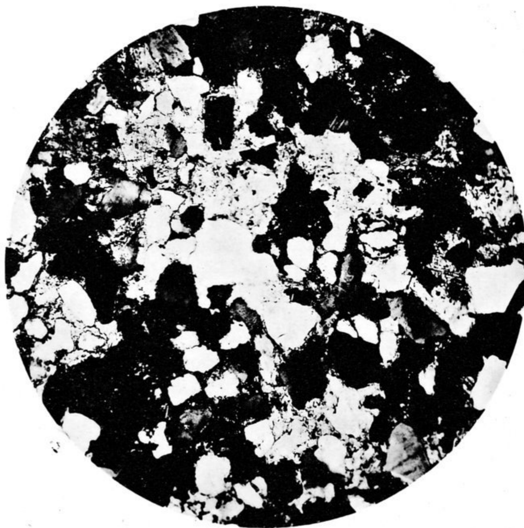
Fig. 5. Die Schlacke (35) 35mal vergr. Sie zeigt die divergentstrahlige Struktur der langen Olivinleisten. Fig. 6. Grauwackenartiger Kalksandstein (72). Eckige und gerundete Körner von Quarz und Feldspat von krist. Calcit zusammengekittet. + Nicols. Vergr. 60:1.
