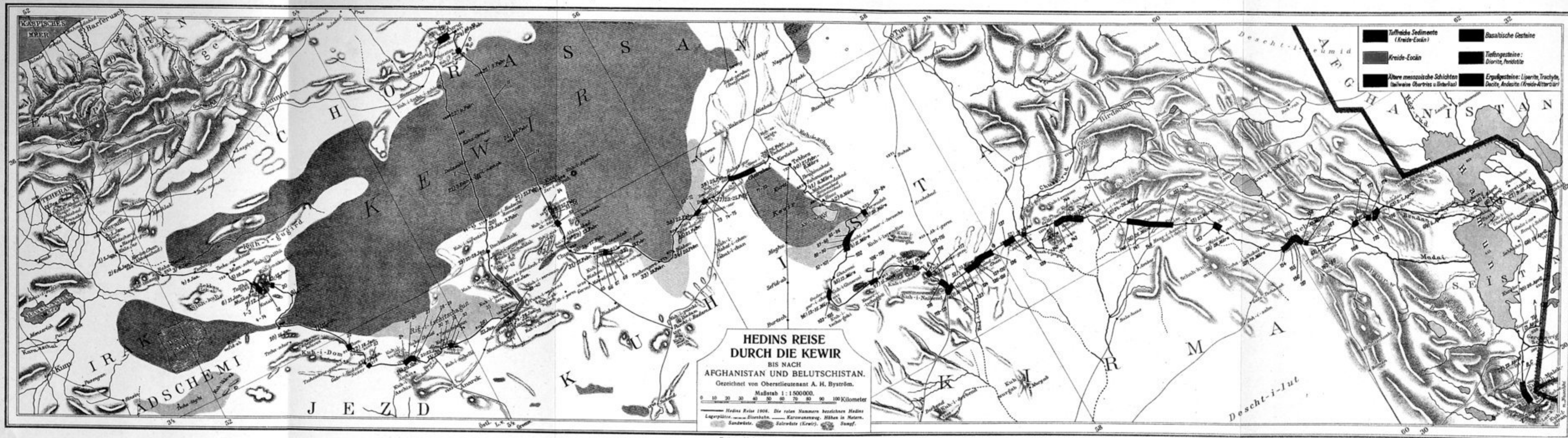
Geologische Karte über die Routenaufnahme Sven Hedins durch Ostpersien. Zusammengestellt von B. Asklund.
