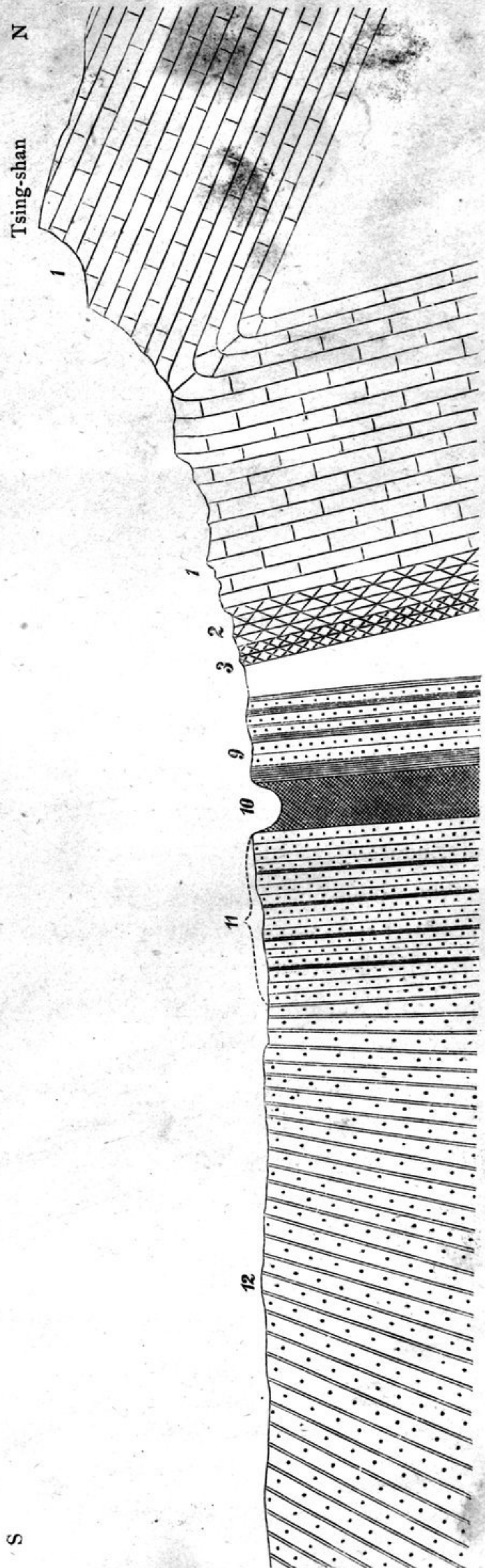
Fig. 58. Profil der Steinkohlenformation westlich von Pai-tau-tszé .
