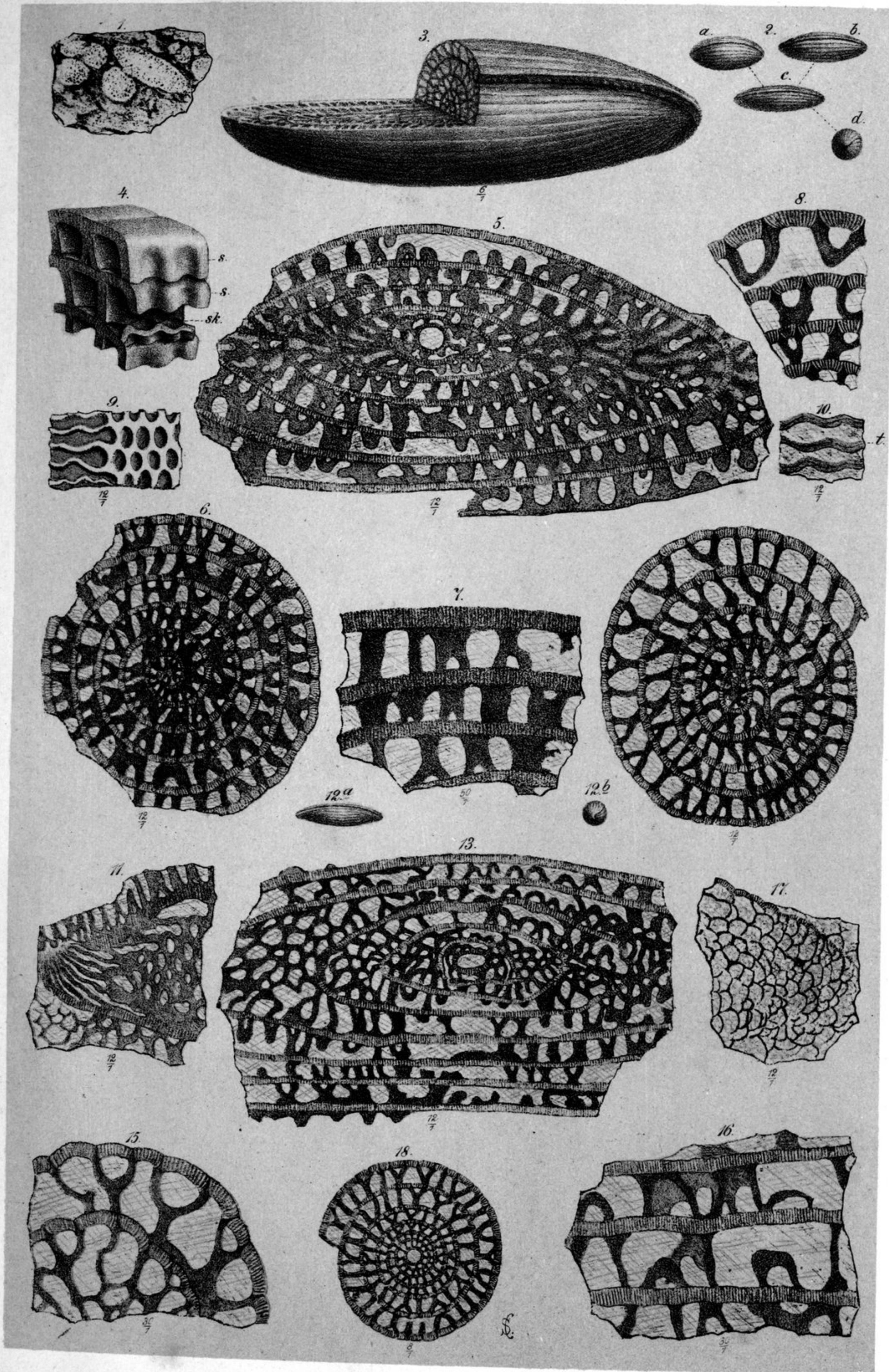
SCHWAGER, CARBON-FORAMINIFEREN.
