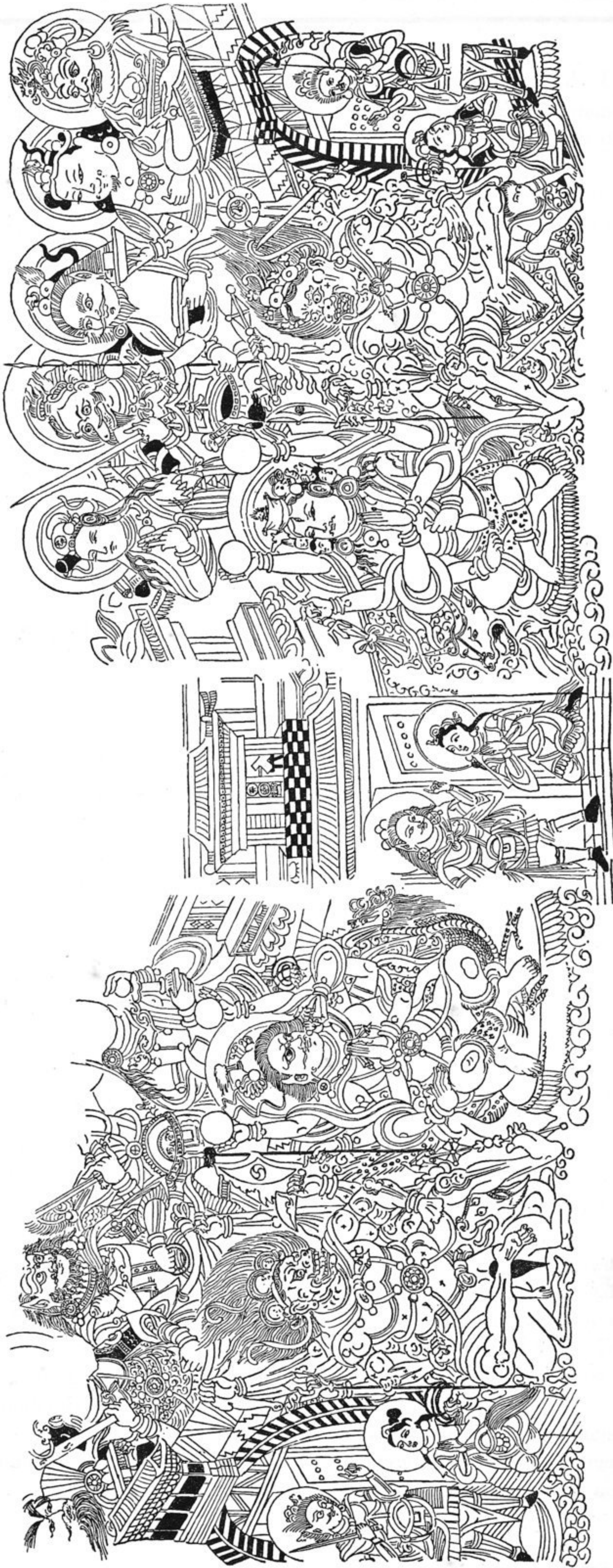
Fig. 75. Darstellung von drei Himmelstoren, bewacht von vierzehn Schutzgöttern vom Sockel einer zerstörten Avalokitesvara-Figur, kleines Tempelchen A vor der Gräbergruppe von Bäcklik, Kultst. S. 229—230.
