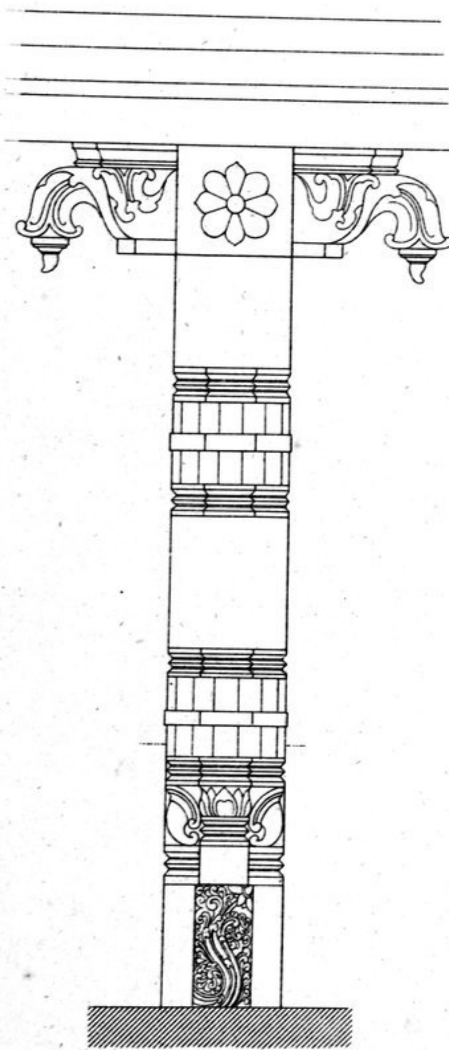
COLUMN E
