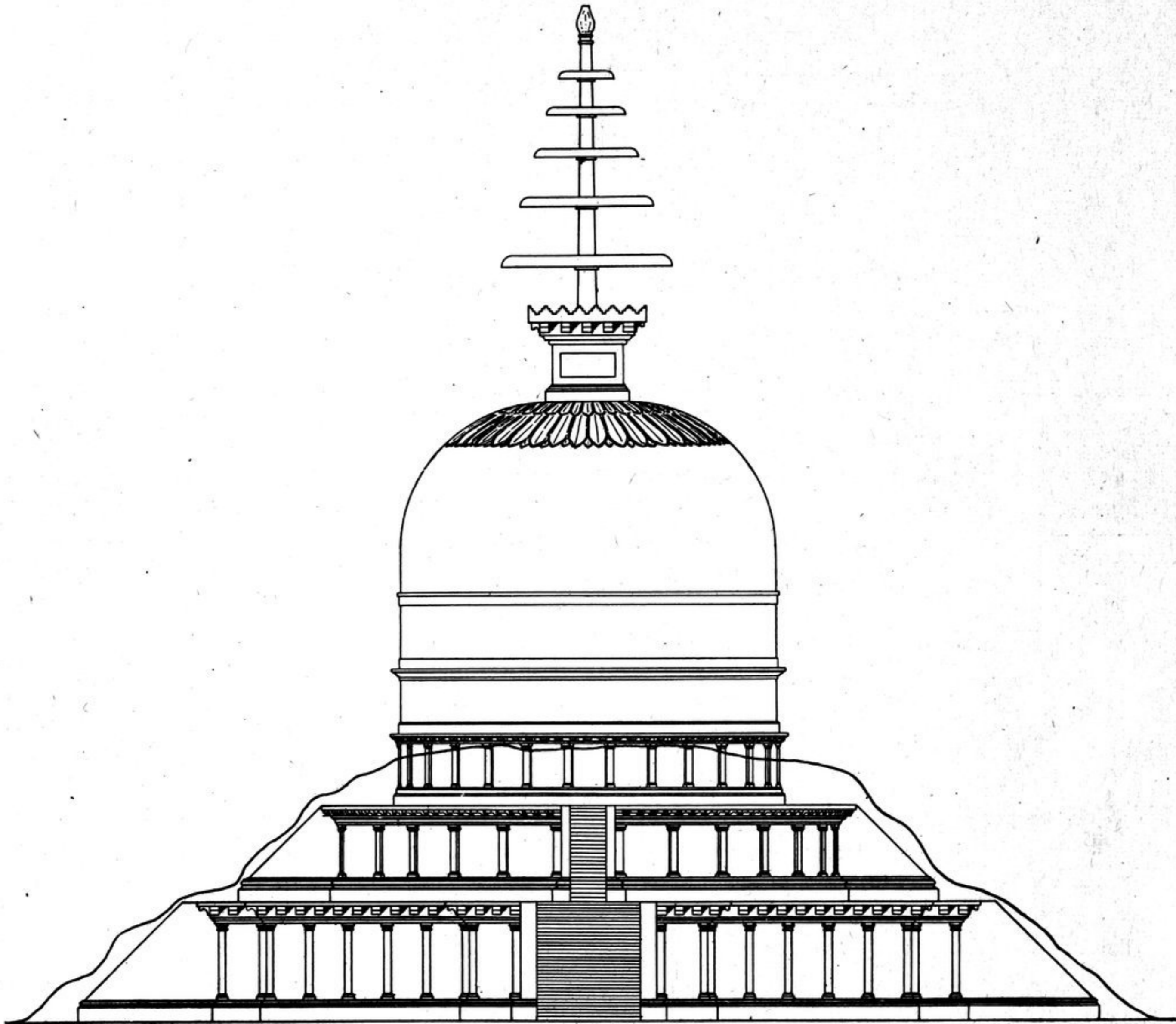
Fig. 24. — ESSAI DE RECONSTITUTION DU TÔP-É-RUSTAM : ÉLÉVATION. (Cf. pl. XXI d, XXIX d, XXX c et XXXII d.)
