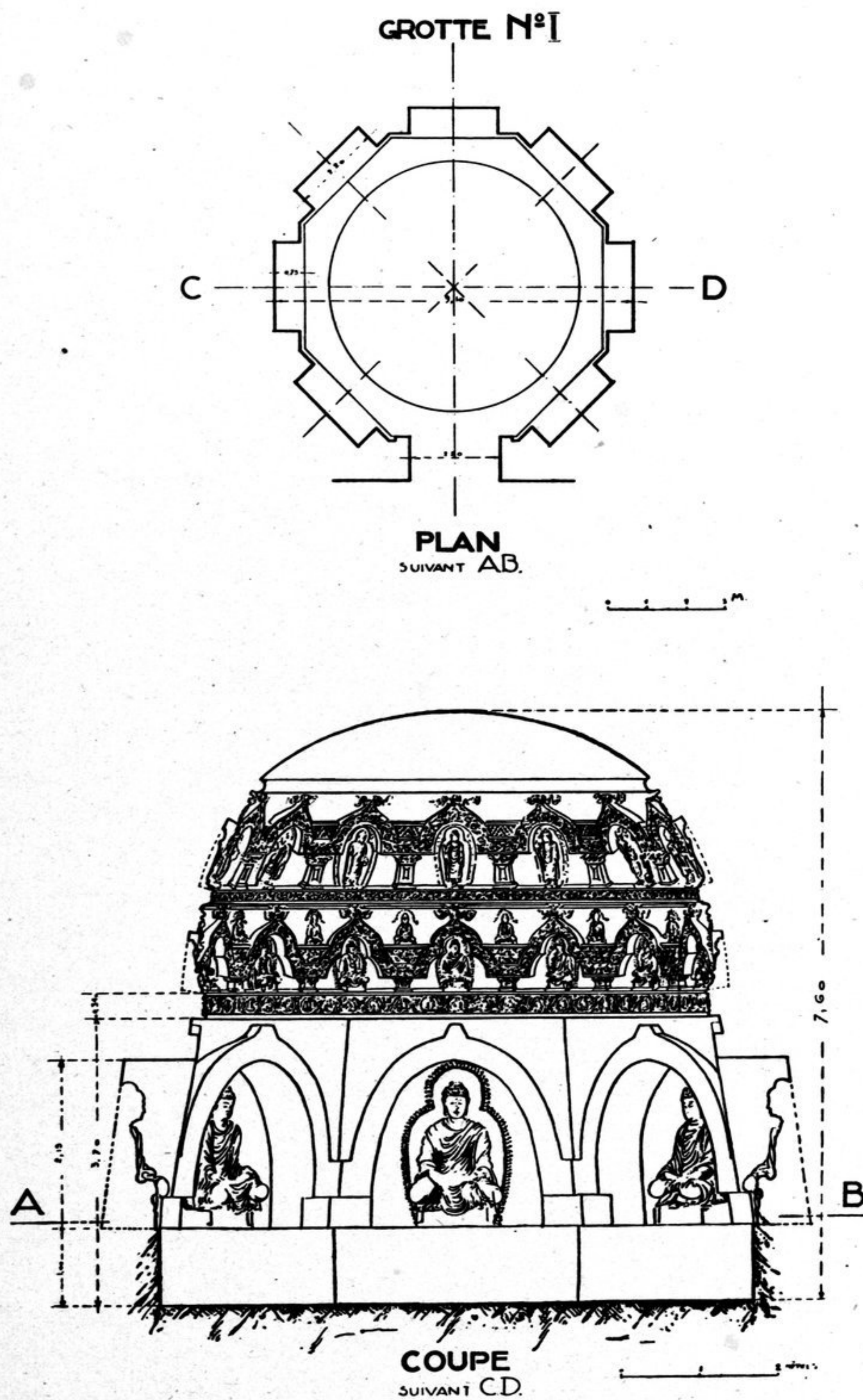
FIG. V. — Grotte I. Plan, coupe et restitution de la décoration modelée de la grotte.
