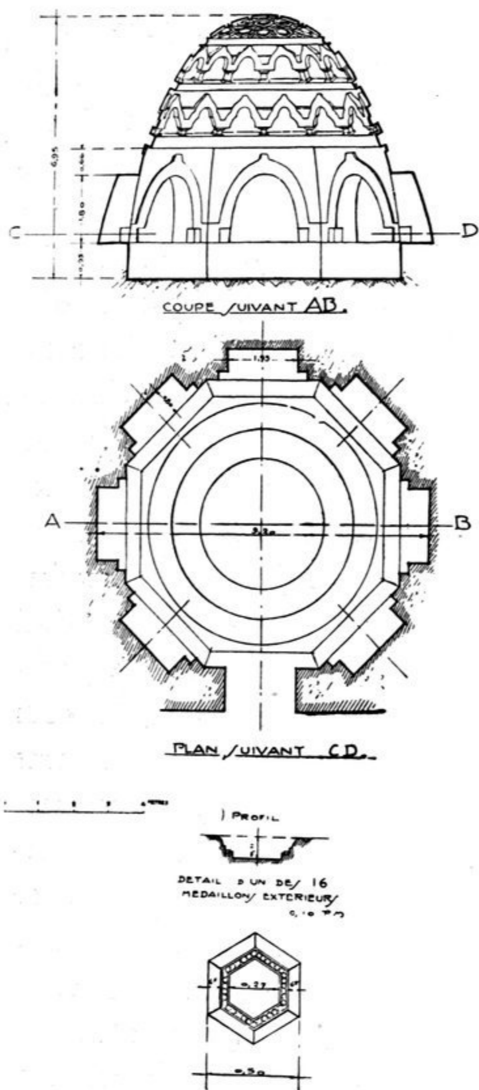
FIG. VI. — Grotte XI. Plan et coupe. Restitution de l'ornementation de la calotte de la coupole.
