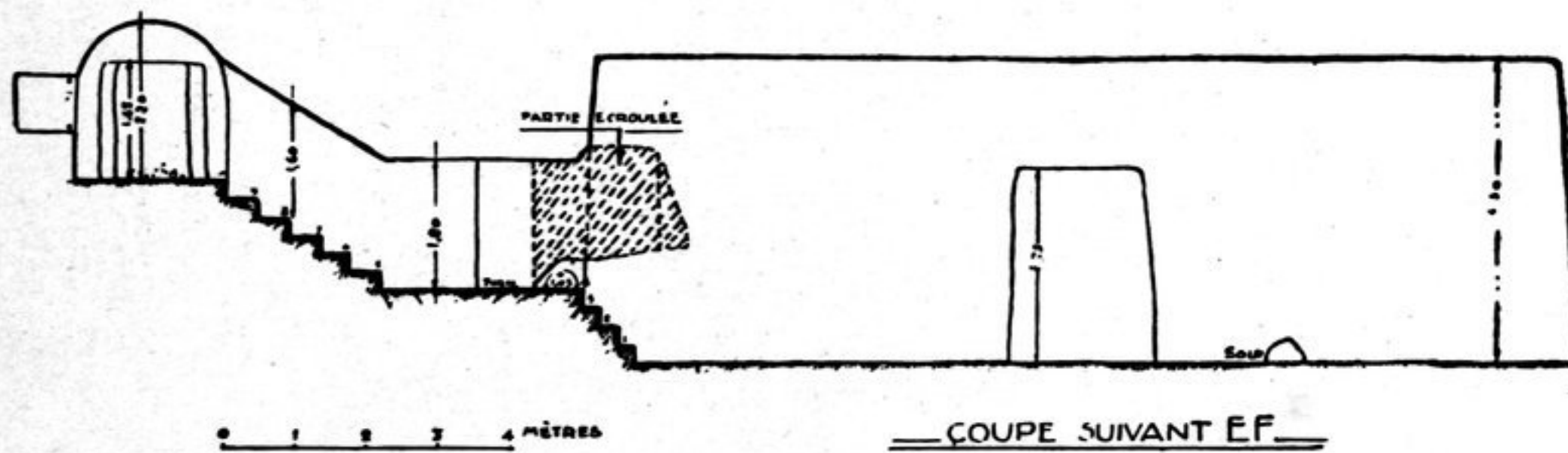
FIG. VII. — Groupe de grottes F. Plan et coupe.
