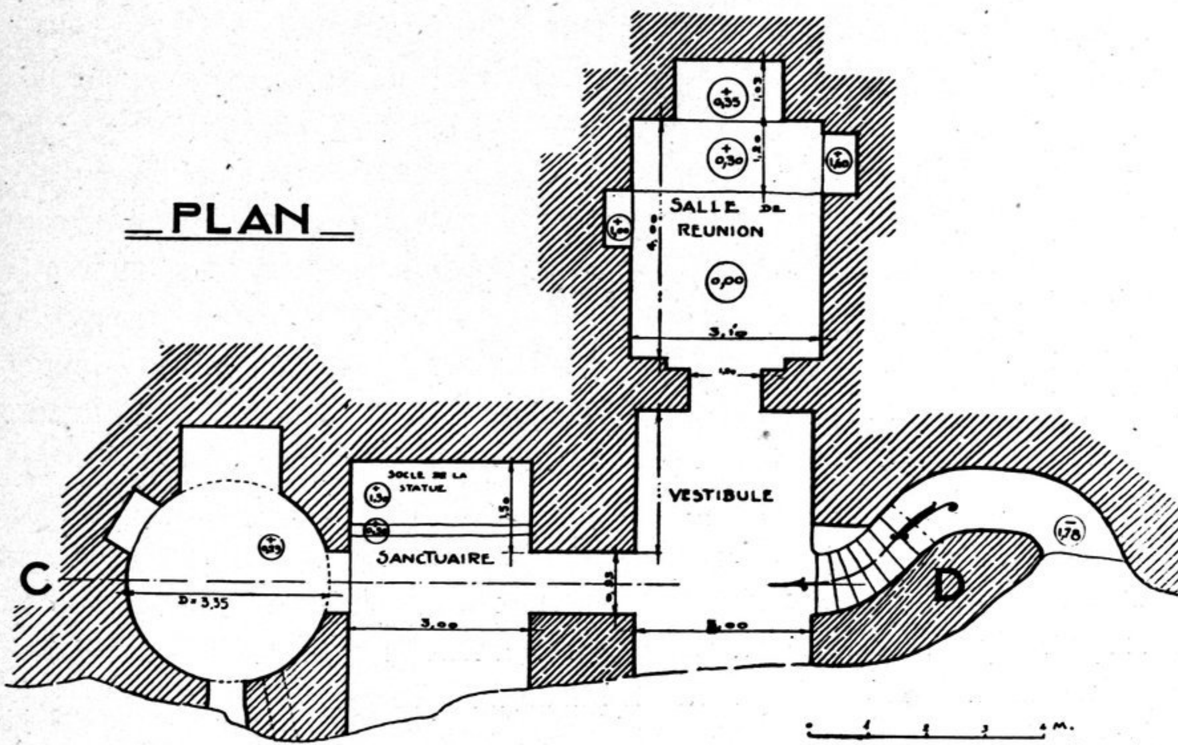
Fig. VIII. — Groupe de grottes XII. Plan et coupe.
