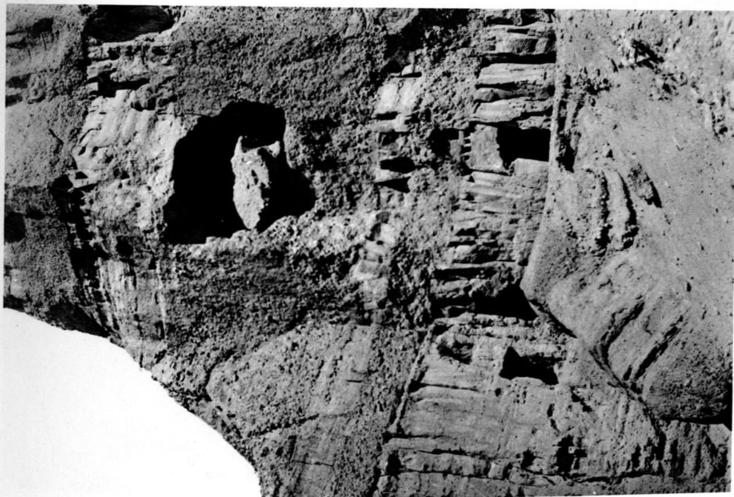
FIG. 49. — ÉTAT DE LA FALAISE A L'OUEST DU GROUPE XII.
