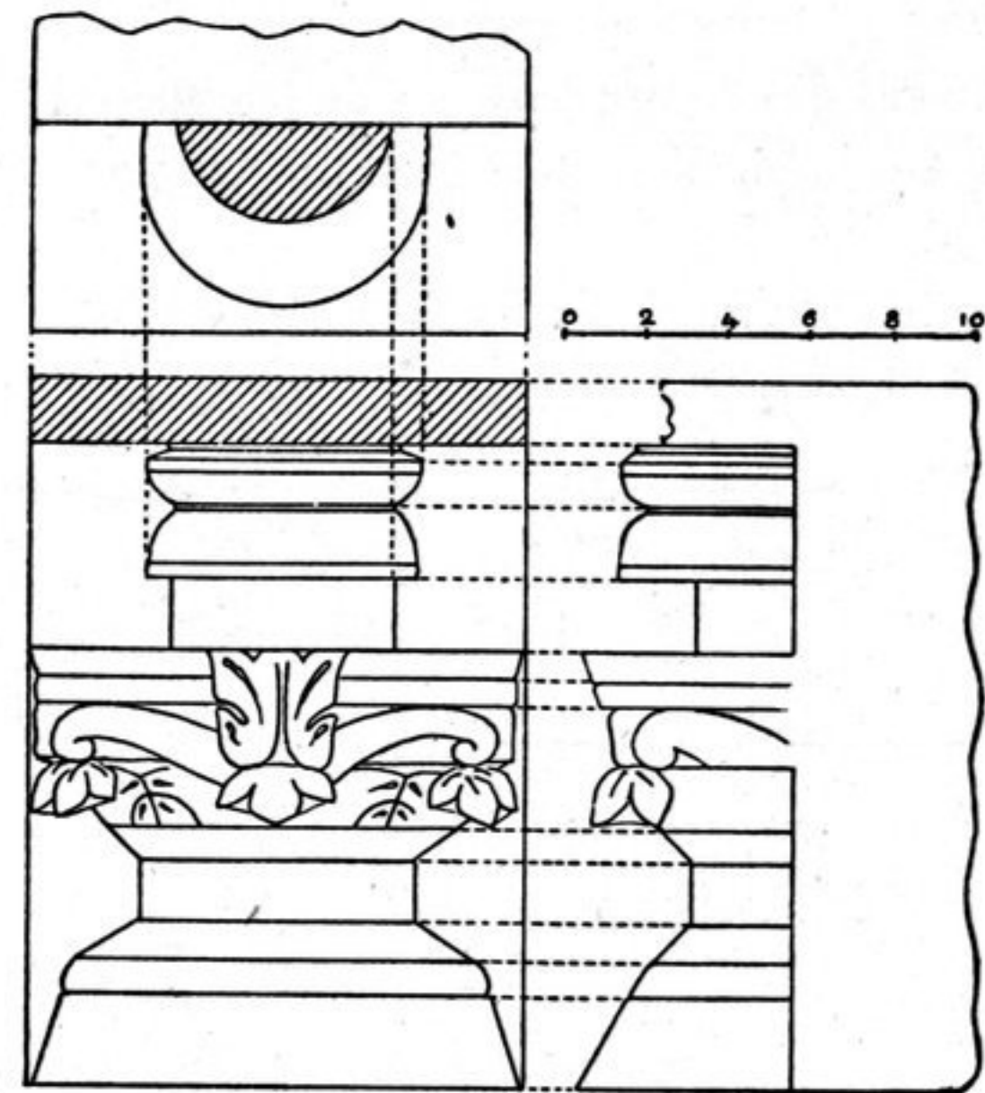
FIG. 10. — Double pilastre, ayant à la partie supérieure, un chapiteau campaniforme simple.
