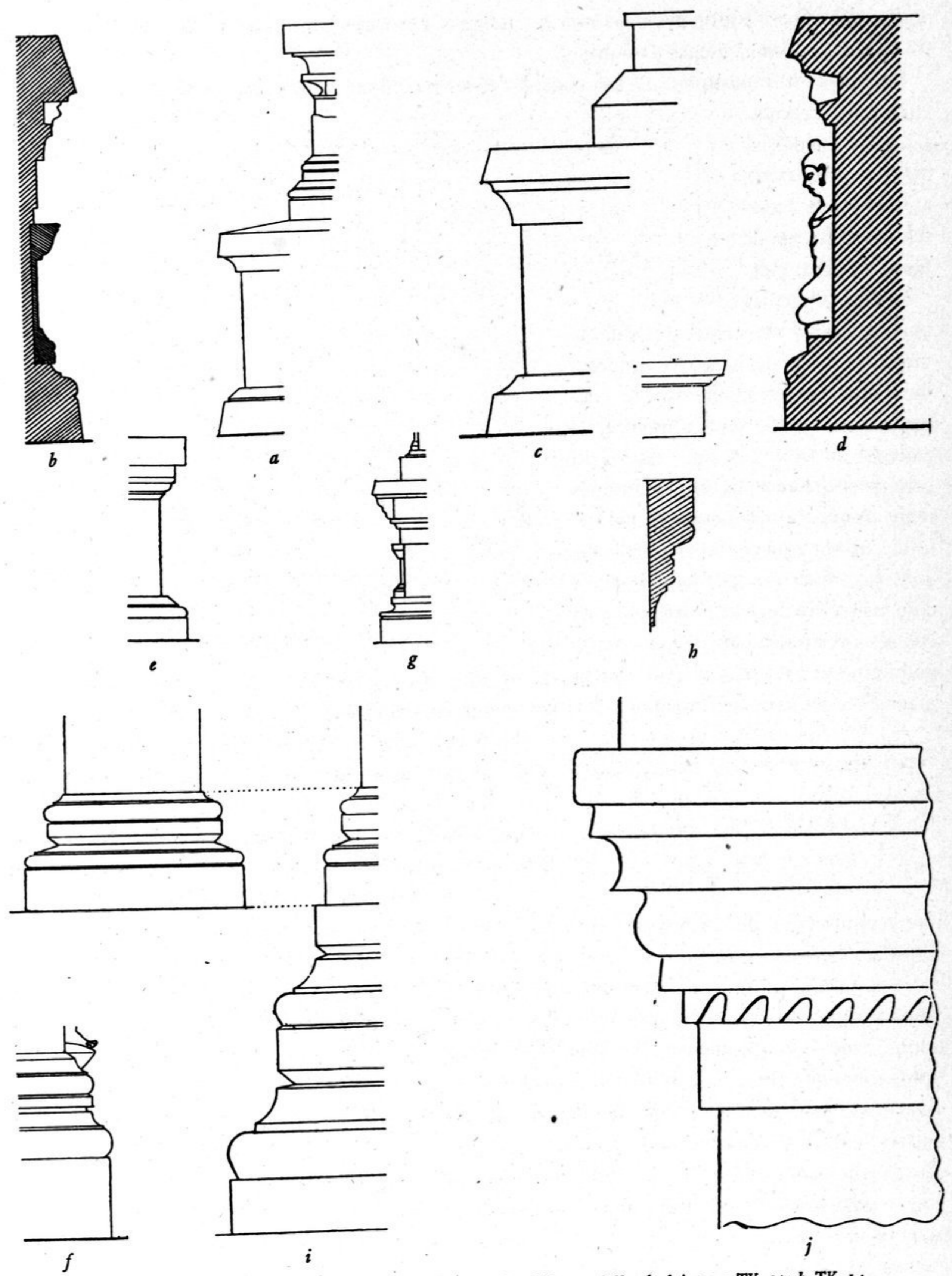
FIG. 14. — Profils de stūpas : a, TK, 88 ; b, B, 12 ; c, TK, 63 ; d, B, 5 ; e, TK, 46 ; f, A, 1 ; g, TK, 14 ; h, TK, 1 ; i, TK, 141 ; j, B, 30.
