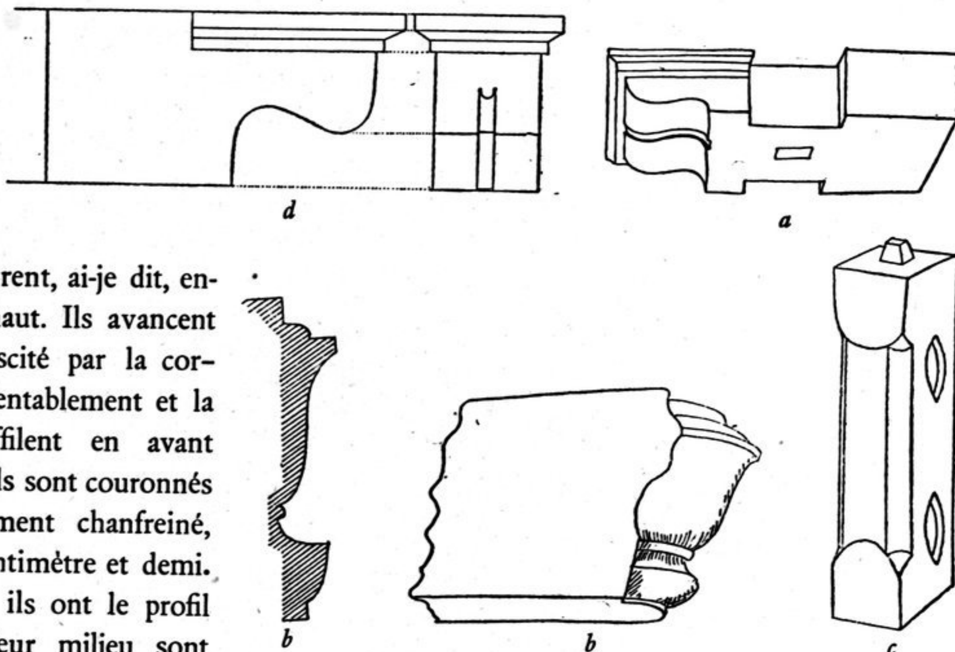
FIG. 15. — Consoles en pierre de TK, 68.
