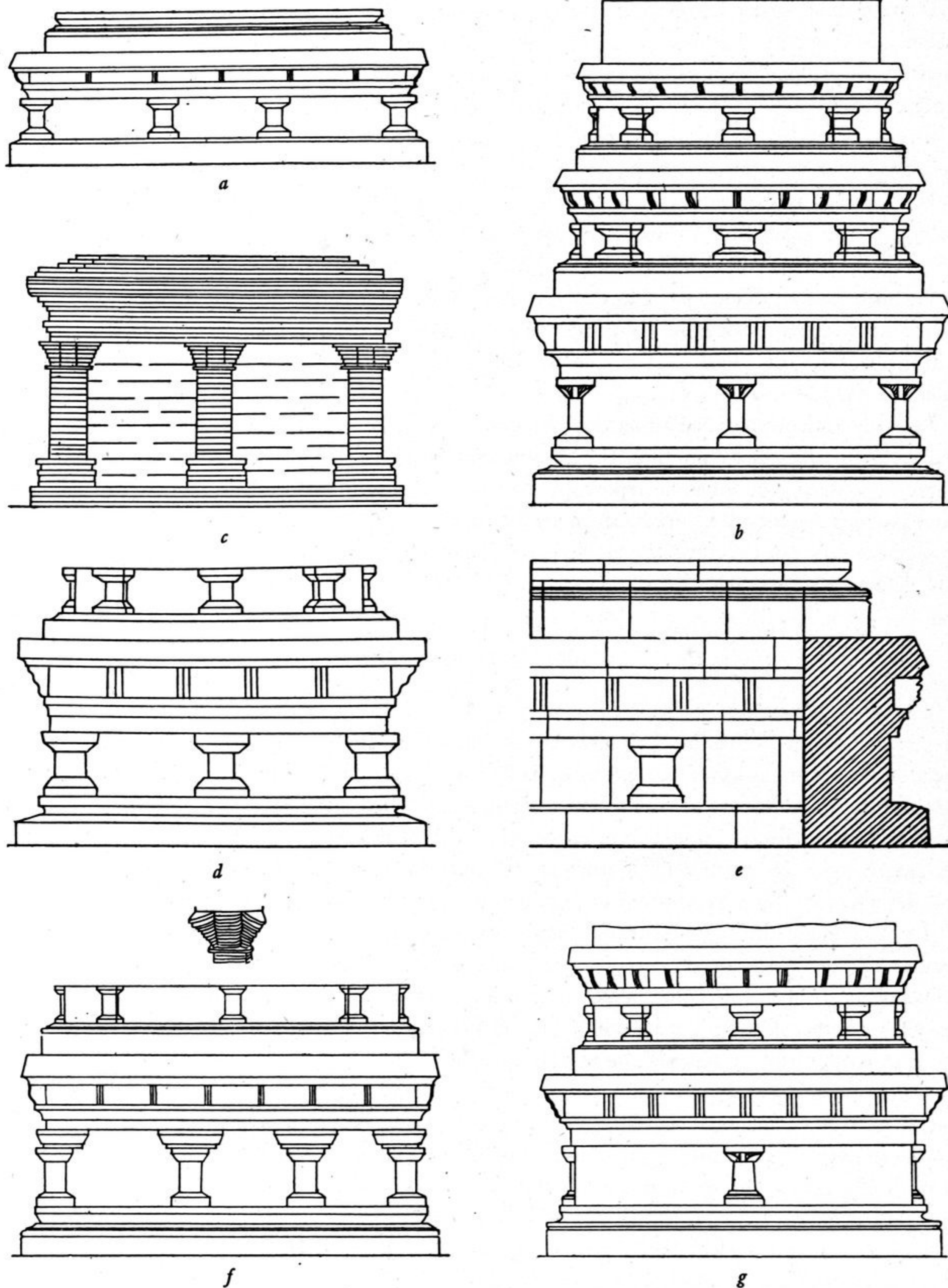
FIG. 29. — Stūpa dépourvus de leur revêtement de stuc, montrant l'appareil et la taille des pierres : a, St. TK, 131, b, st. TK, 134 (pierres de taille) ; c, st. TK, 41 (schiste) ; d, st. TK, 14 ; e, st. B, 21 : assemblage de pierres de taille ; f, st. TK, 117 bis ; g, st. TK, 15 (pierres de taille).
