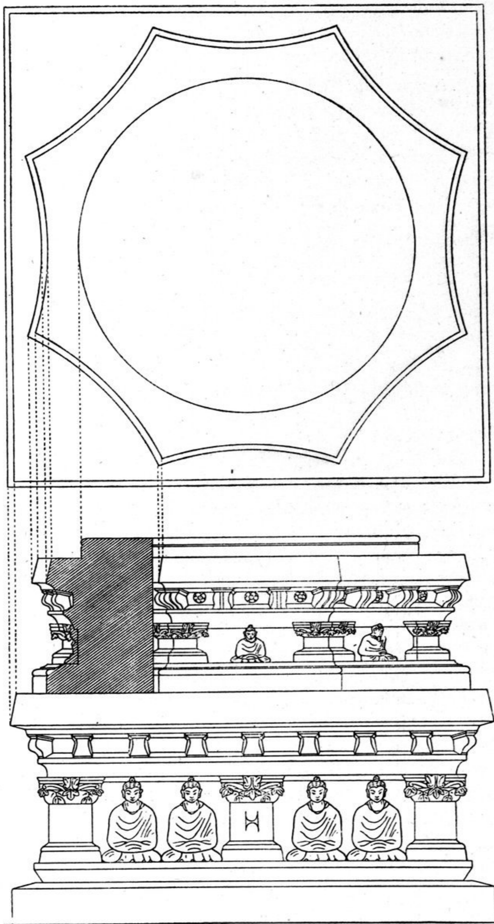
FIG. 89. — Façade du st. TK, 121 (Éch. 1/10).
