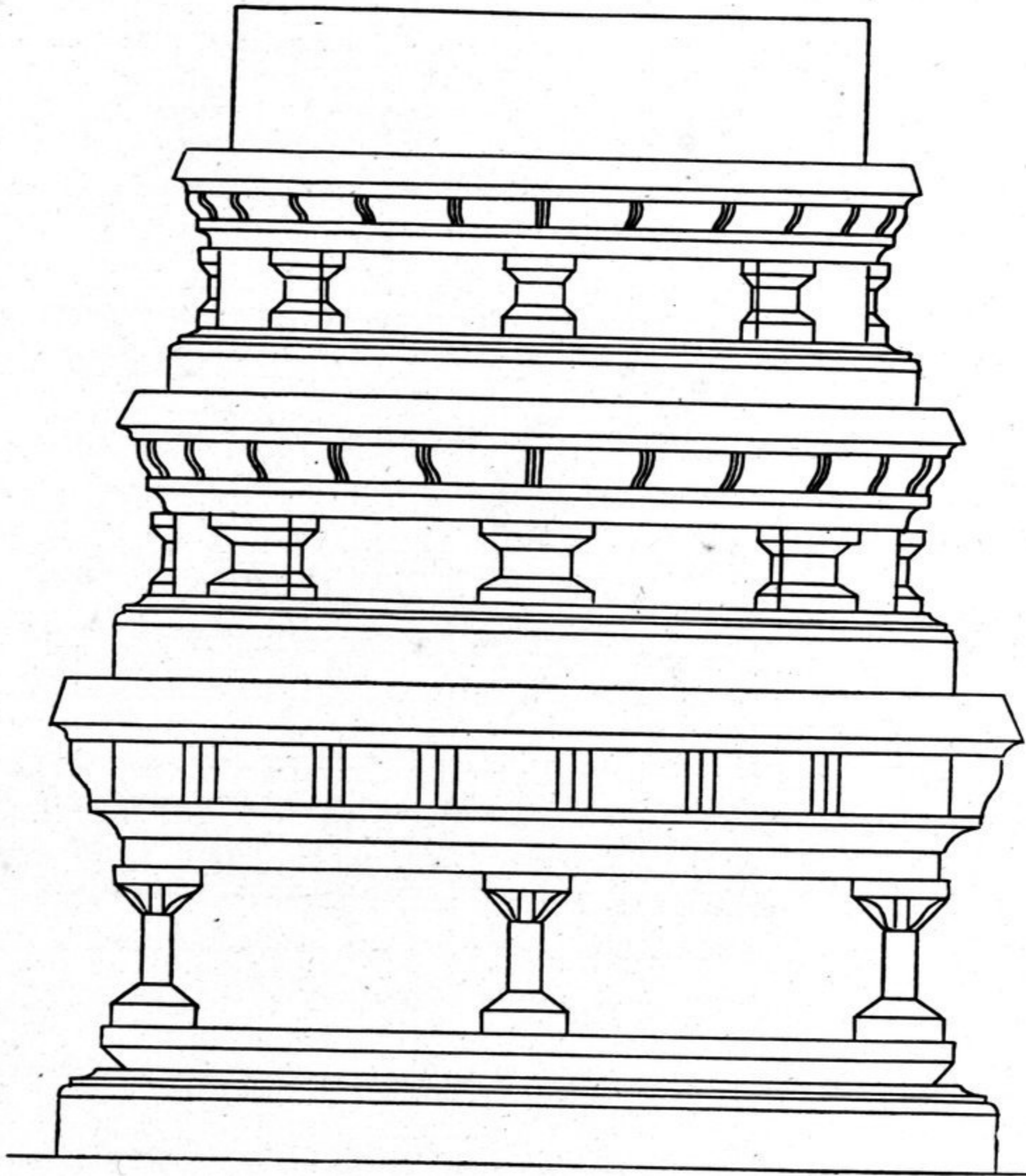
FIG. 94. — St. TK, 134 dépourvu de son revêtement de stuc (Éch. 1/10).
