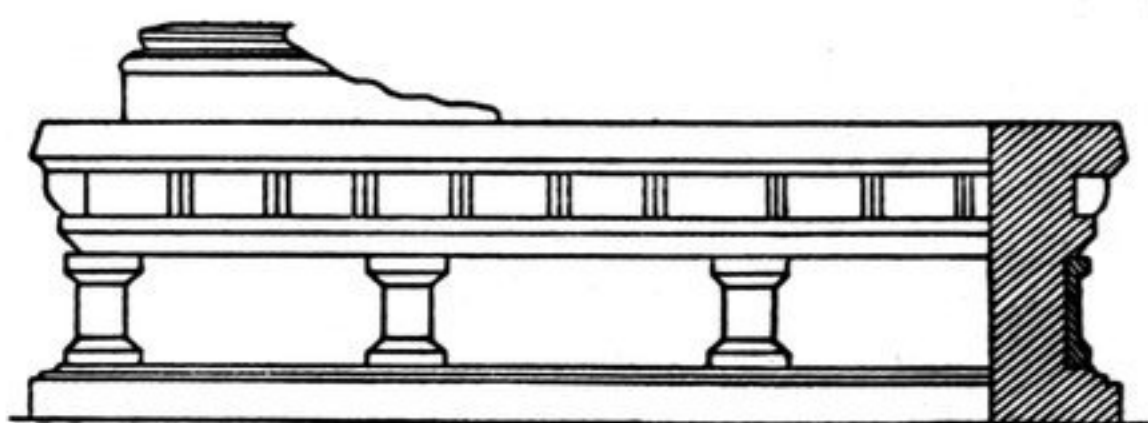
FIG. 95. — Restitution du st. TK, 136 (Éch. 1/20).
