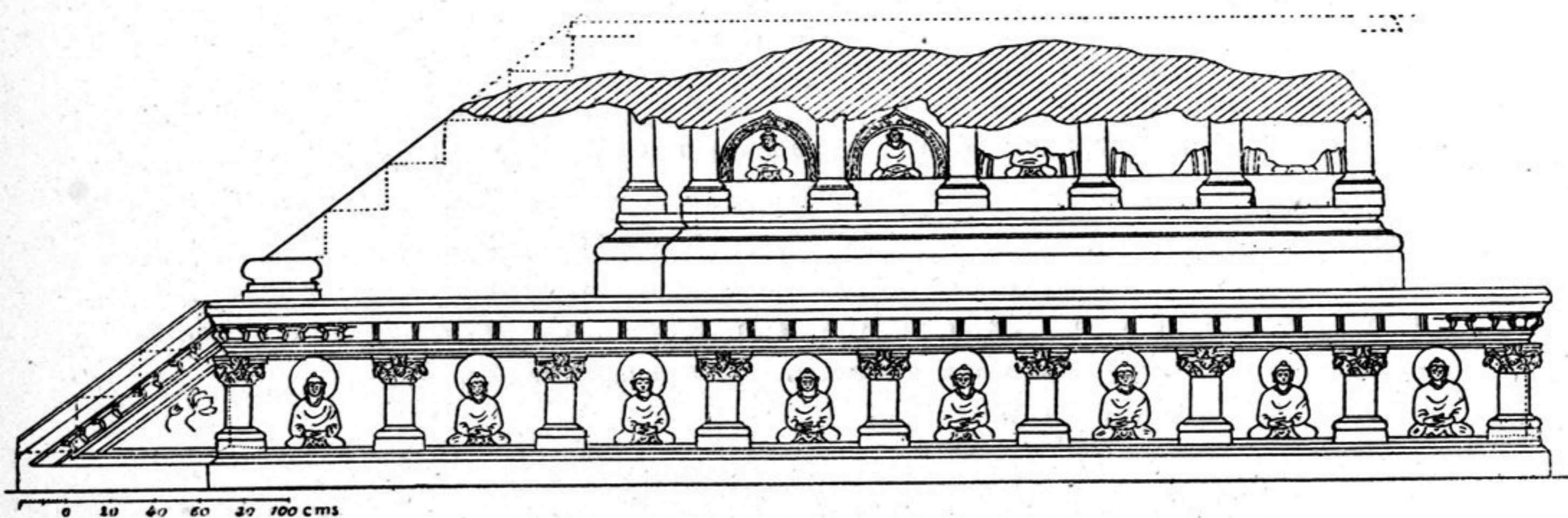
FIG. 113. — Façade du groupe de stūpa K, 43.
