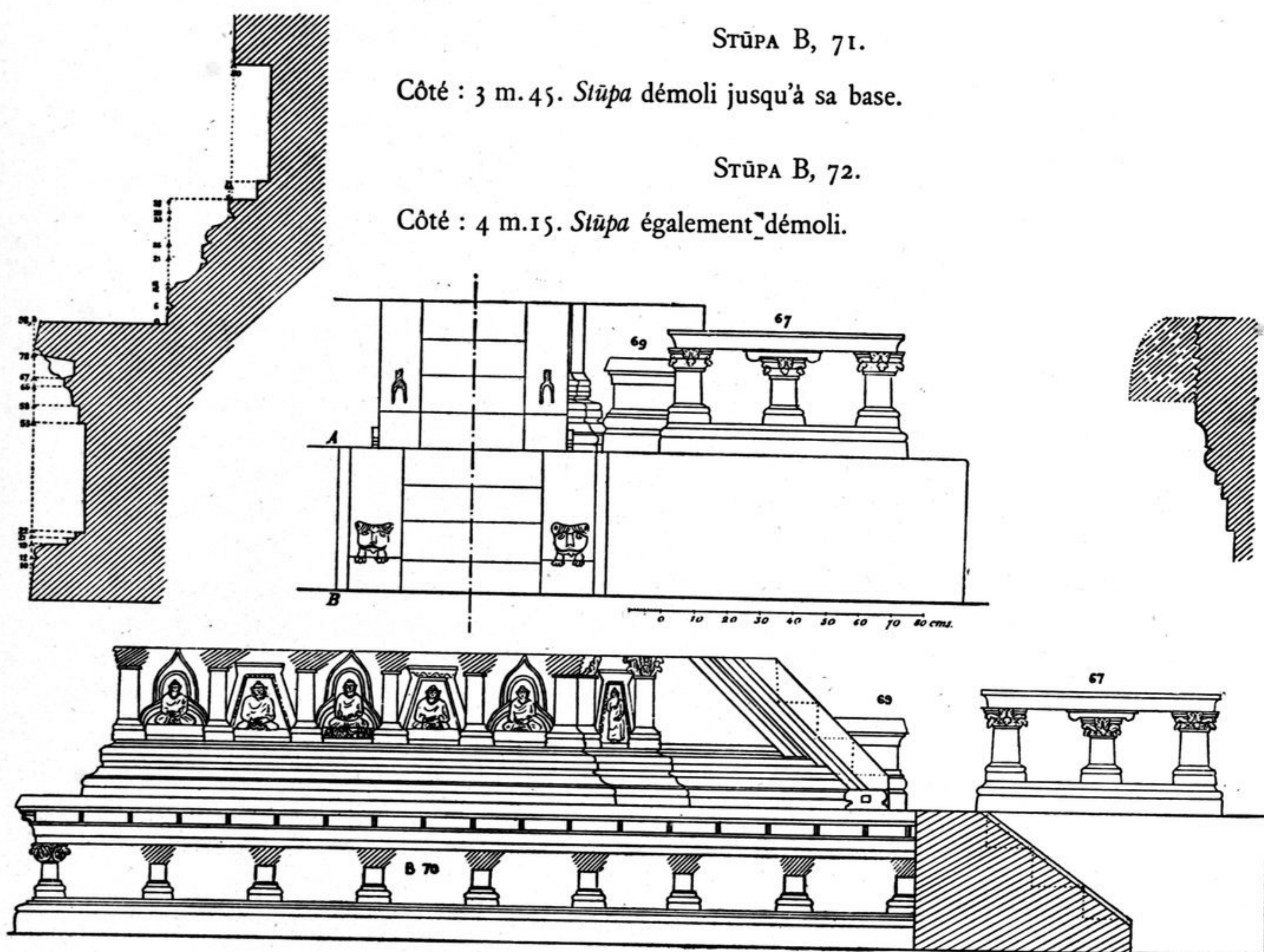
FIG. 150. — Façade SW. du st. B, 70 ; l'escalier inférieur est en coupe. En haut, les escaliers et les stūpa 67 et 69 édifiés sur la plate-forme. A droite, profil de l'entablement de l'escalier ; à gauche, profil du stūpa B, 70 et de sa plate-forme.
