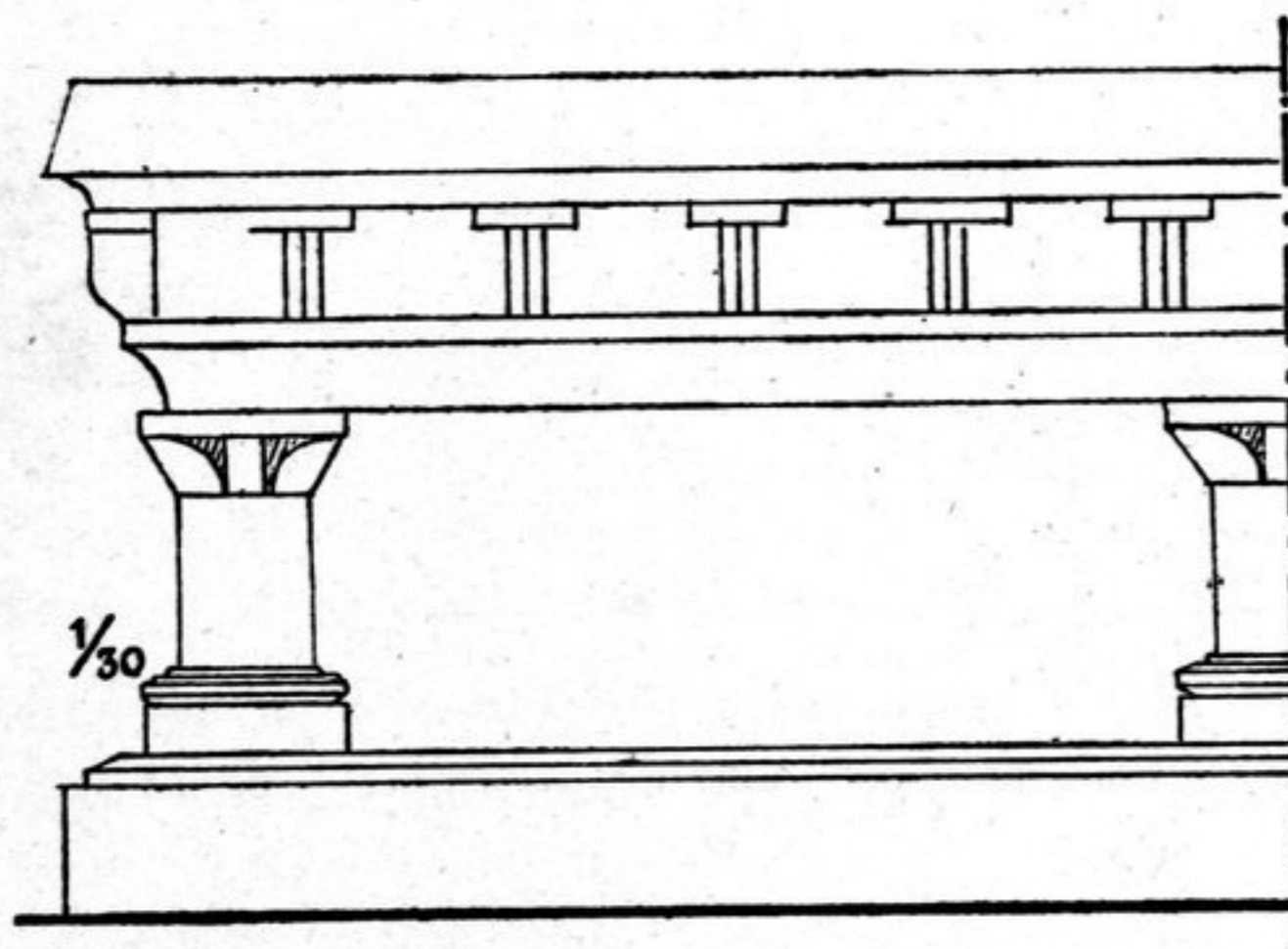
FIG. 186. — Restitution de la façade S. du st. A, 11.
