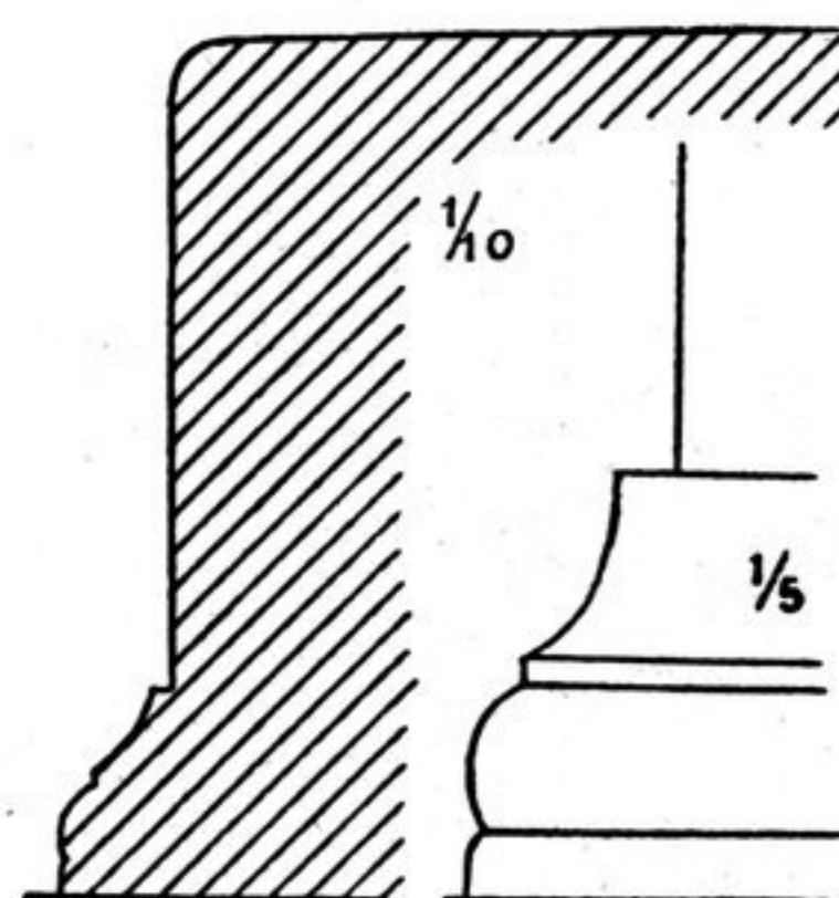
FIG. 196. — Base du st. D, 11.
