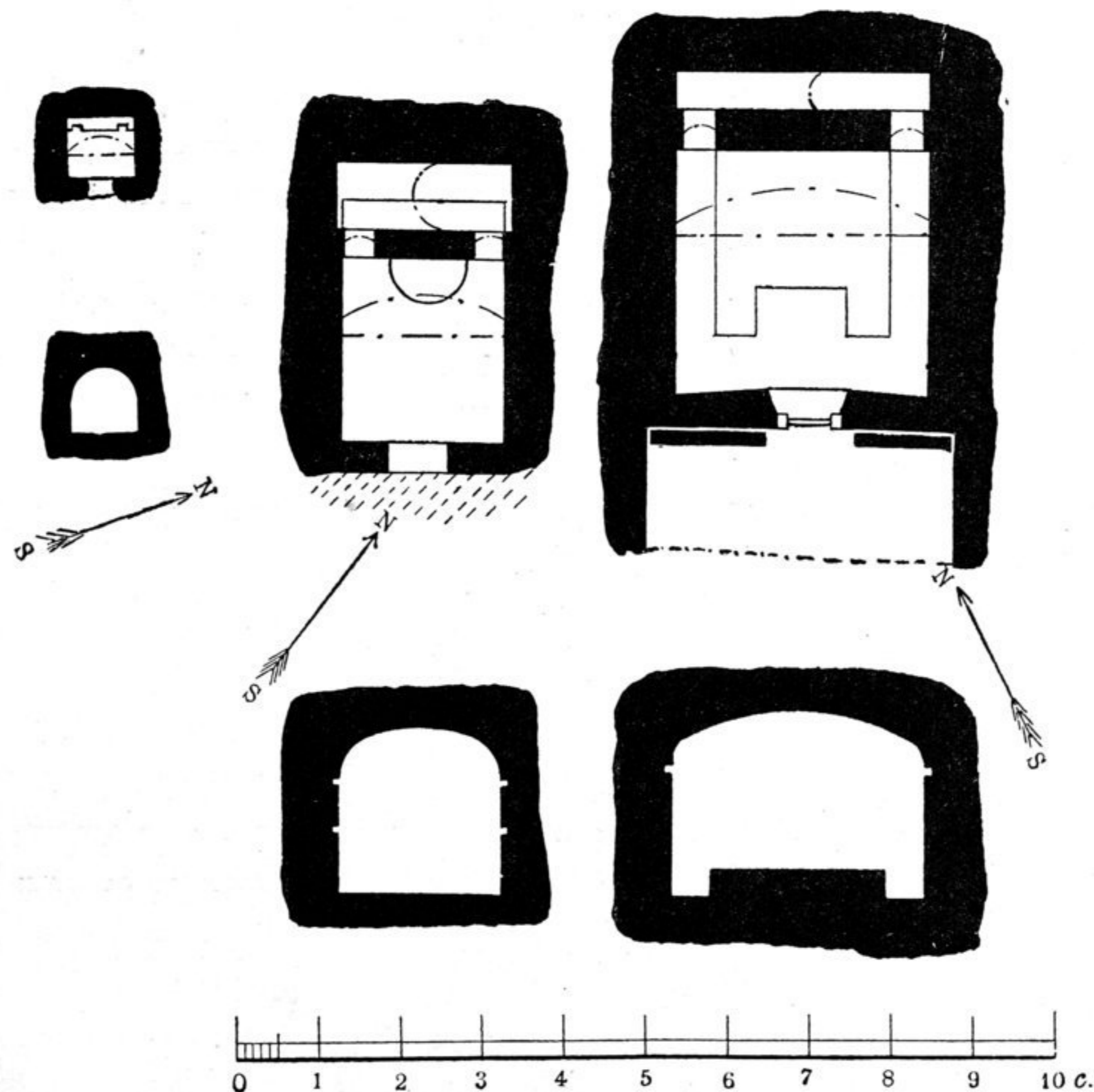
15. Планъ и поперечный разрѣзъ пещеръ №№ 8, 9, 10. Масштабъ 1 сажень = 1 сантиметру.
