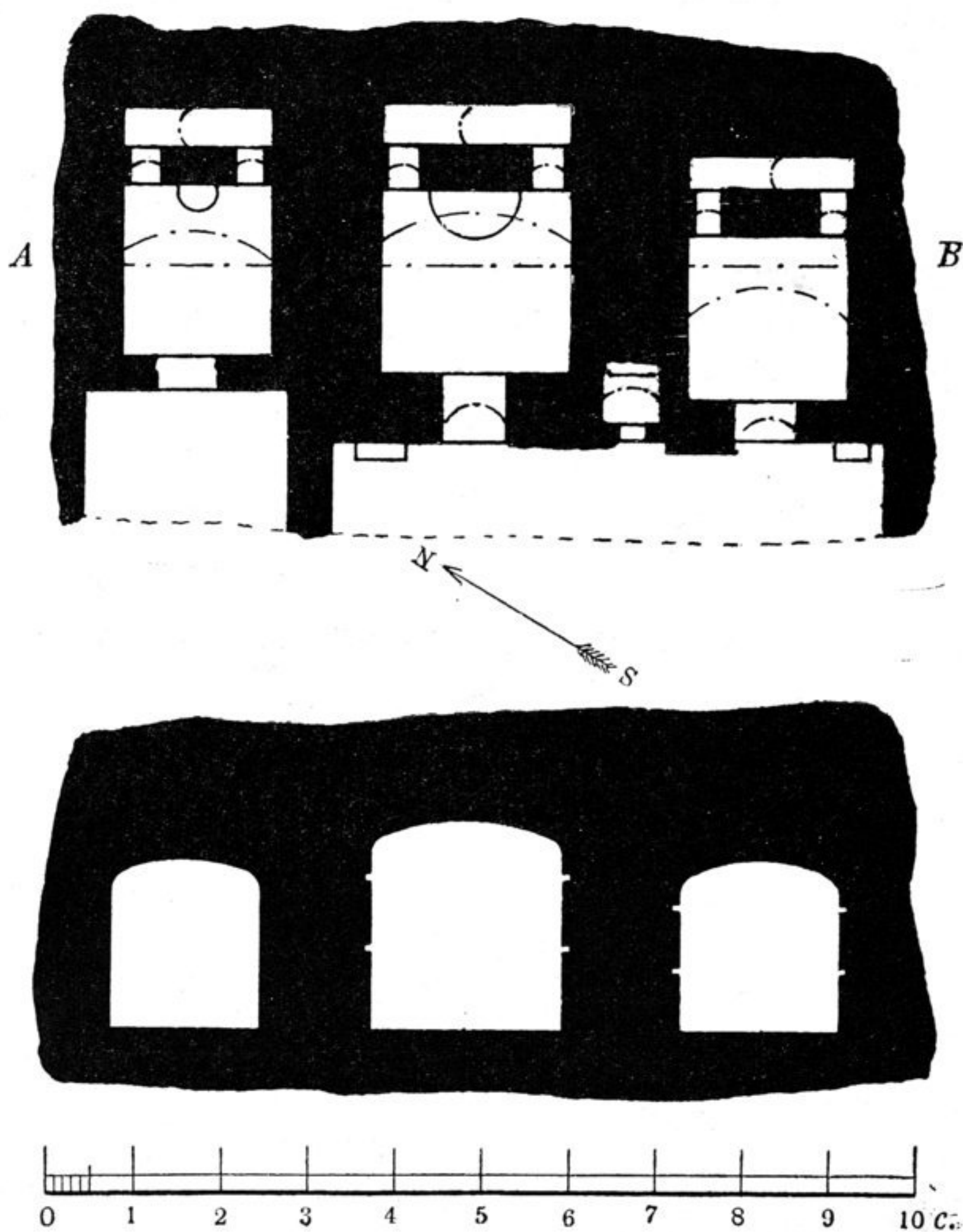
16. Планъ и поперечный разрѣзъ пещеръ №№ 5 и 6.
