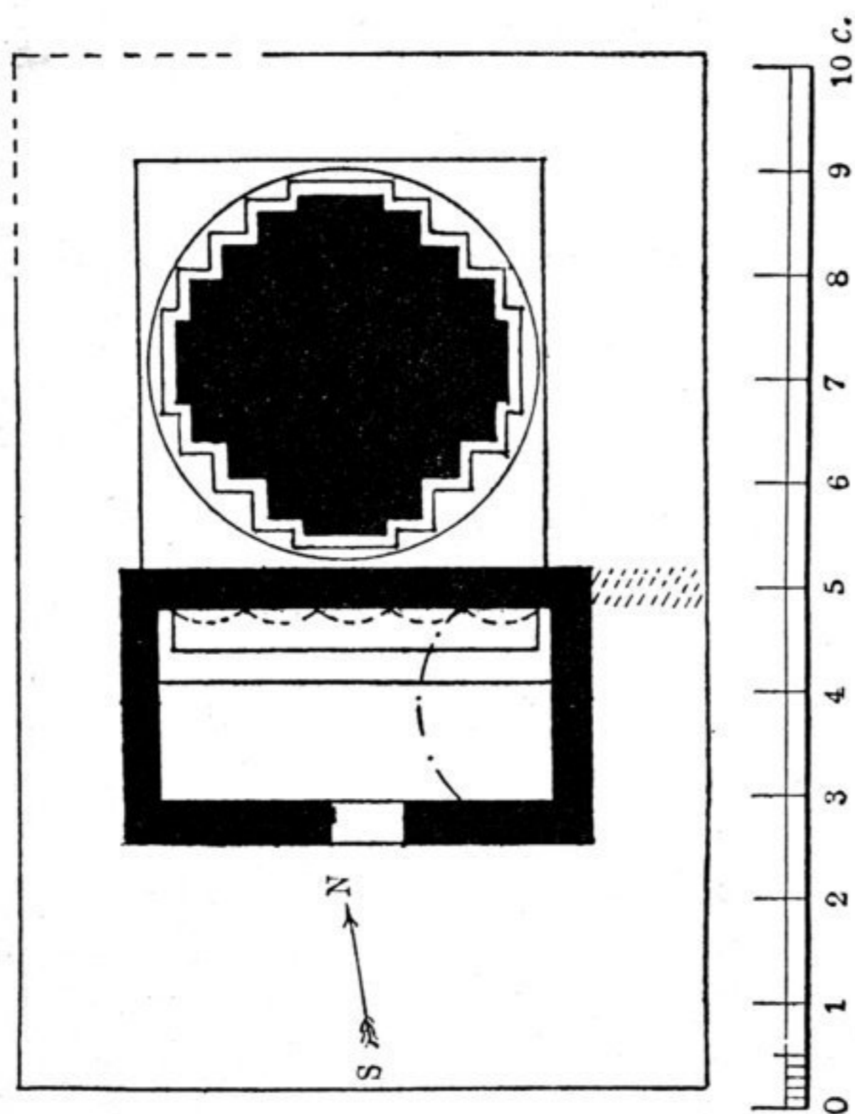
29. Планъ зданія Z въ Идикут-шари.
