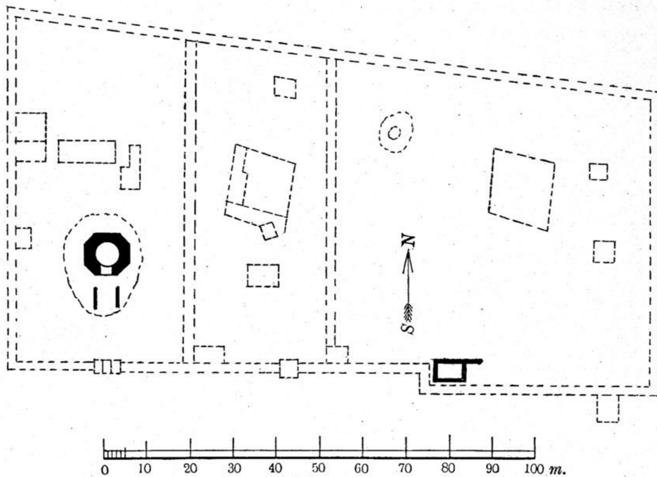
53. Схематическій планъ сѣверной части мѣстности Мин-тен-ата.
