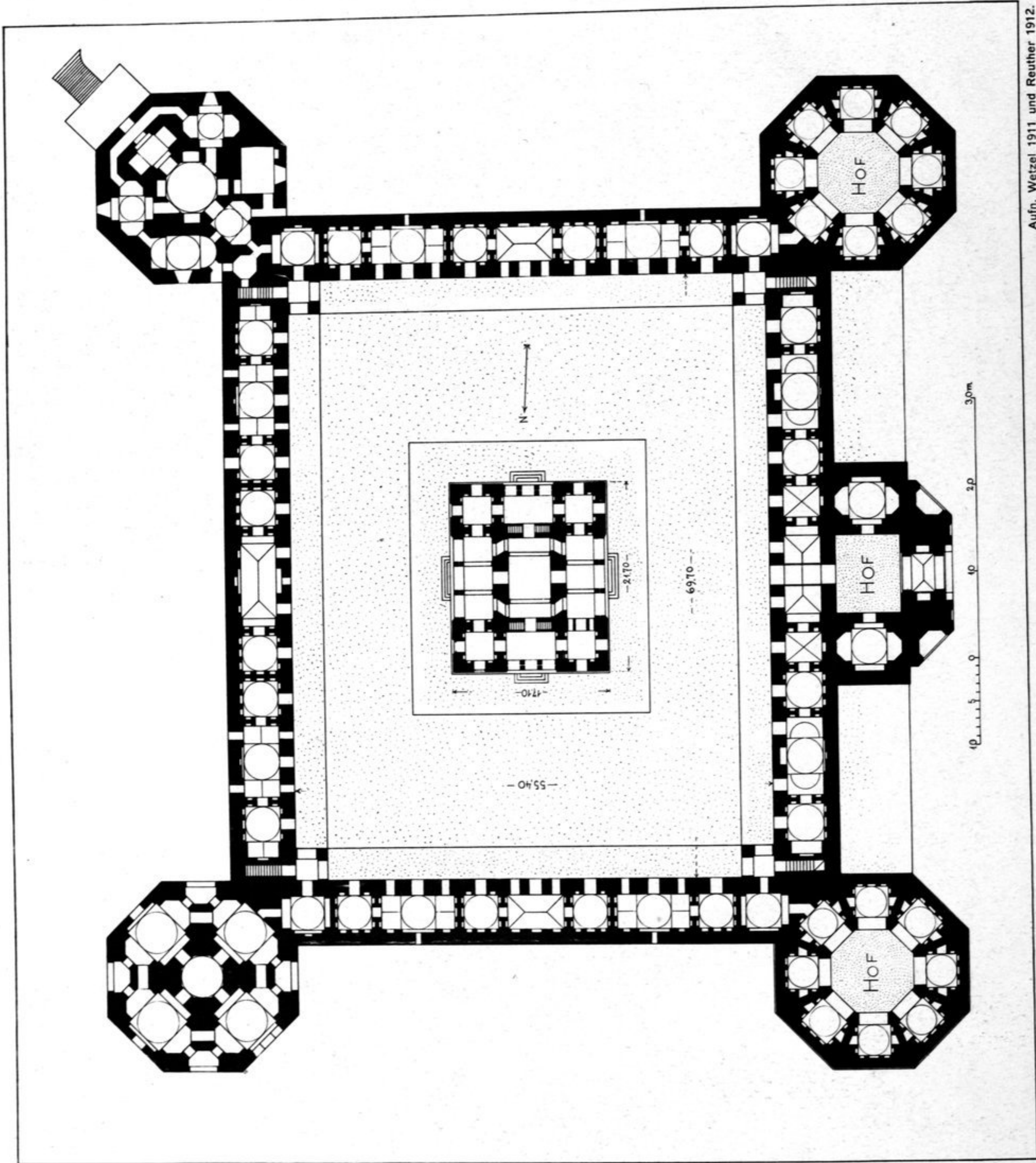
Grundriss des Erdgeschosses.
