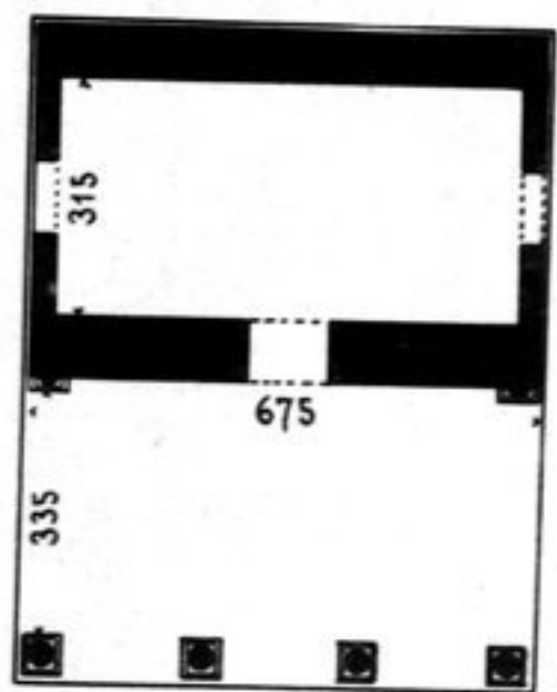
b Grundriss der zweiten Baradari (von Süden gerechnet)
