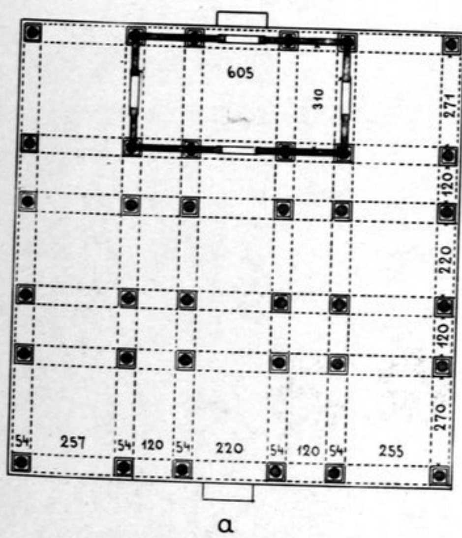
Grundriss der mittelsten Baradari
