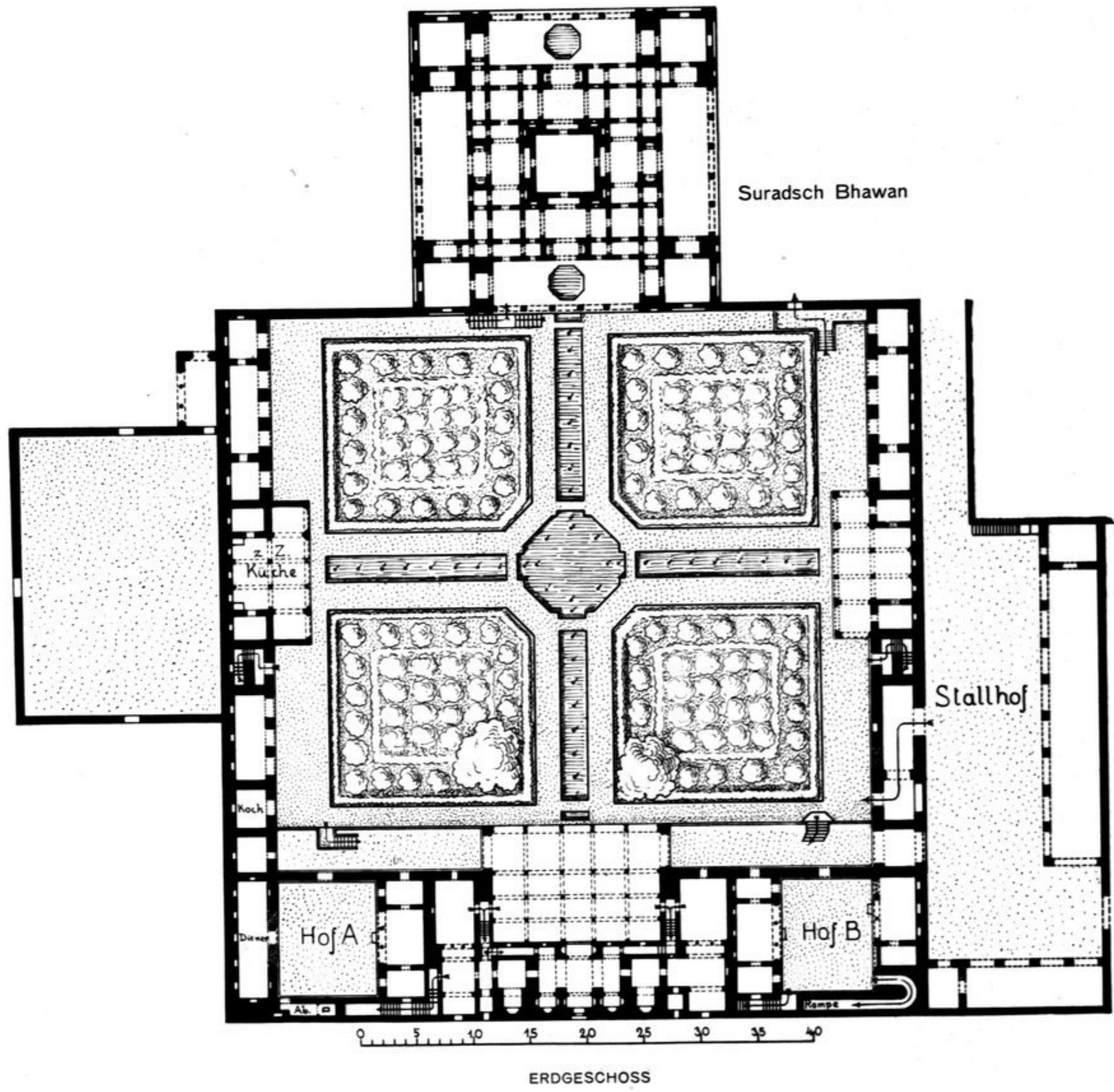
Grundrisse des Hardeo Bhawan und Suradsch Bhawan.
