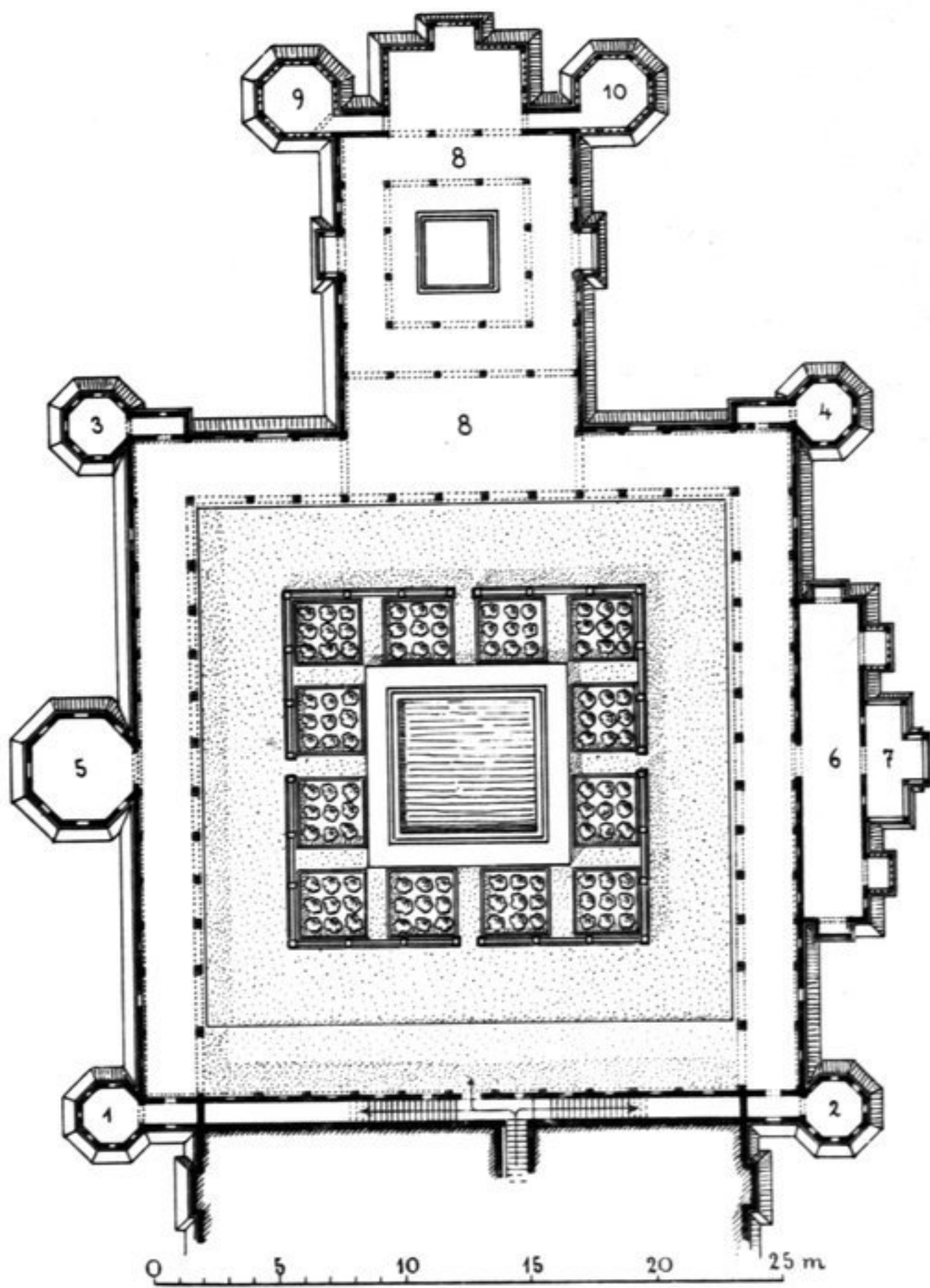
Bari Mahal. Grundriss des Gartengeschosses.
