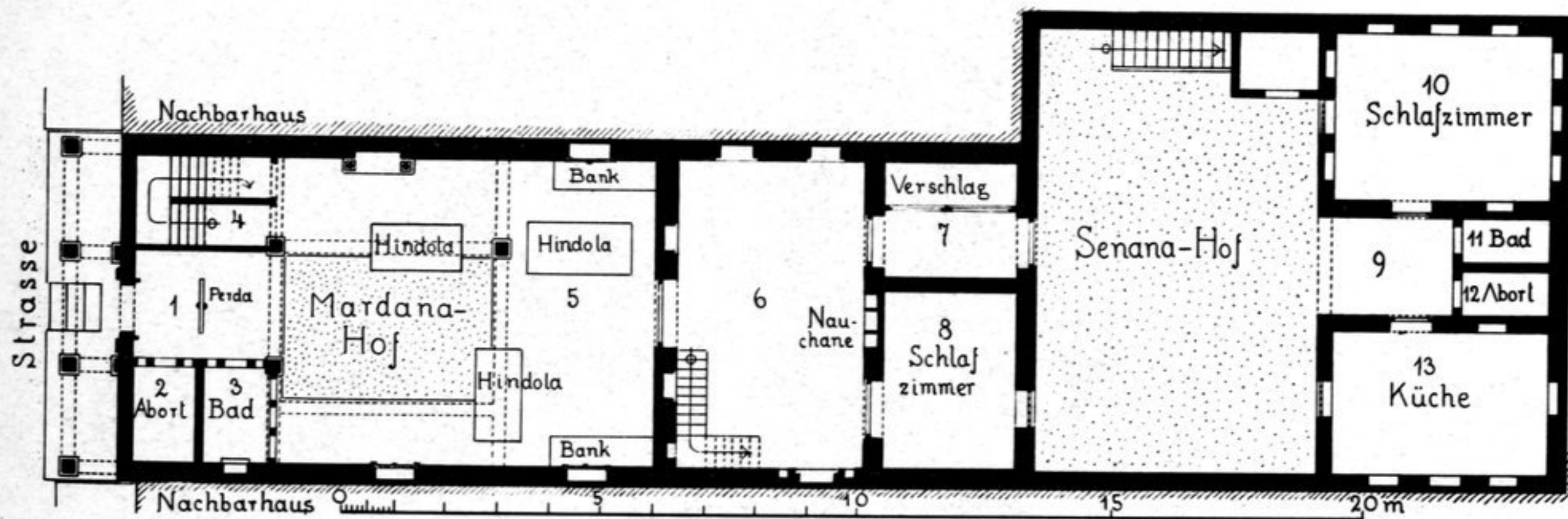
Erdgeschoss
