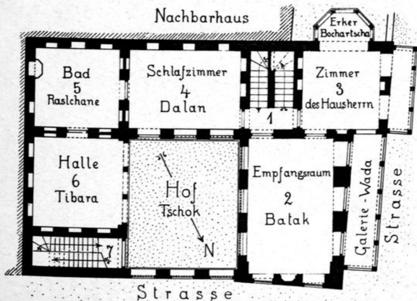
1. Obergeschoss
