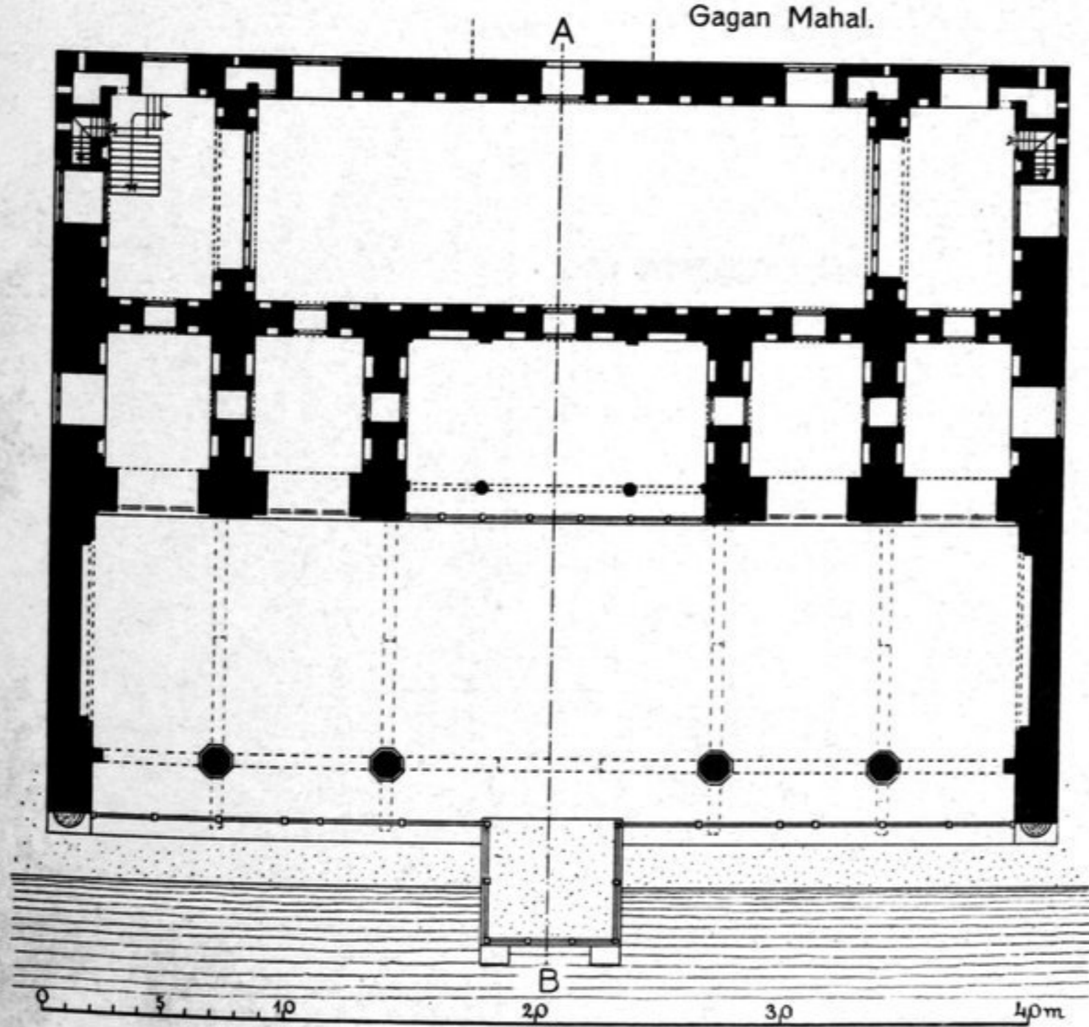
Asar Mahal. Grundriss.
