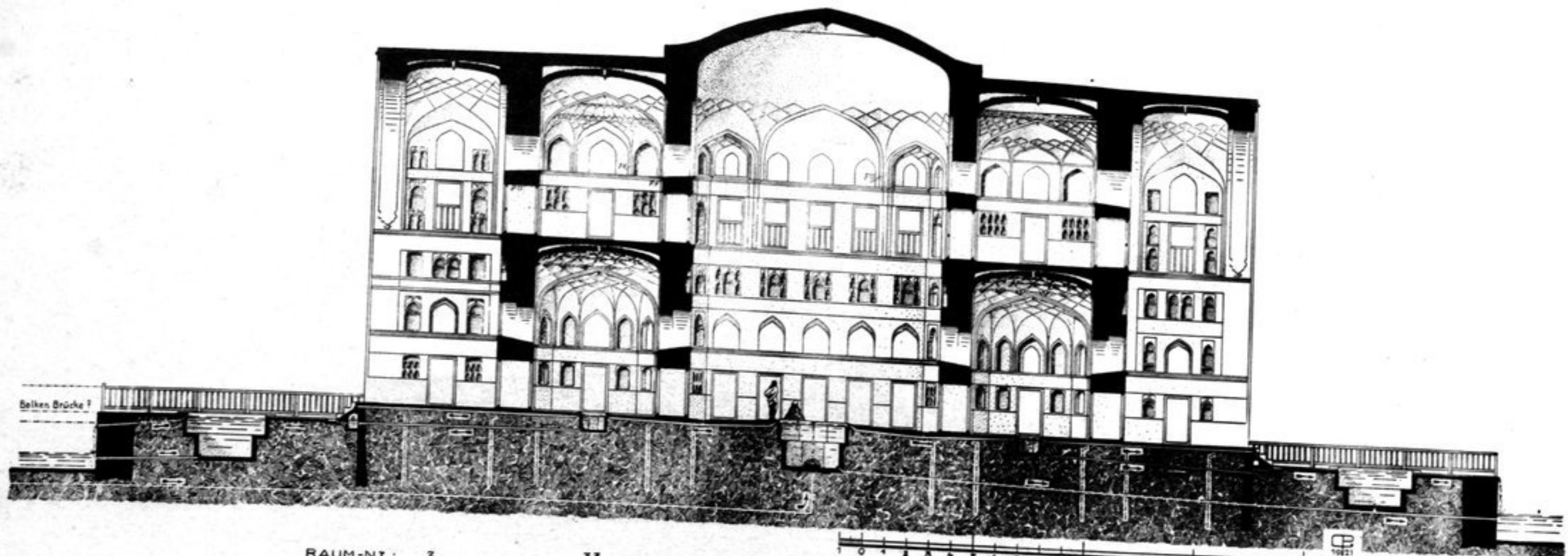
RAUM-Nr.: 3 33 8 13 40 18 25 20 m Mittelschnitt Nord-Süd, Ansicht gegen Ost.
