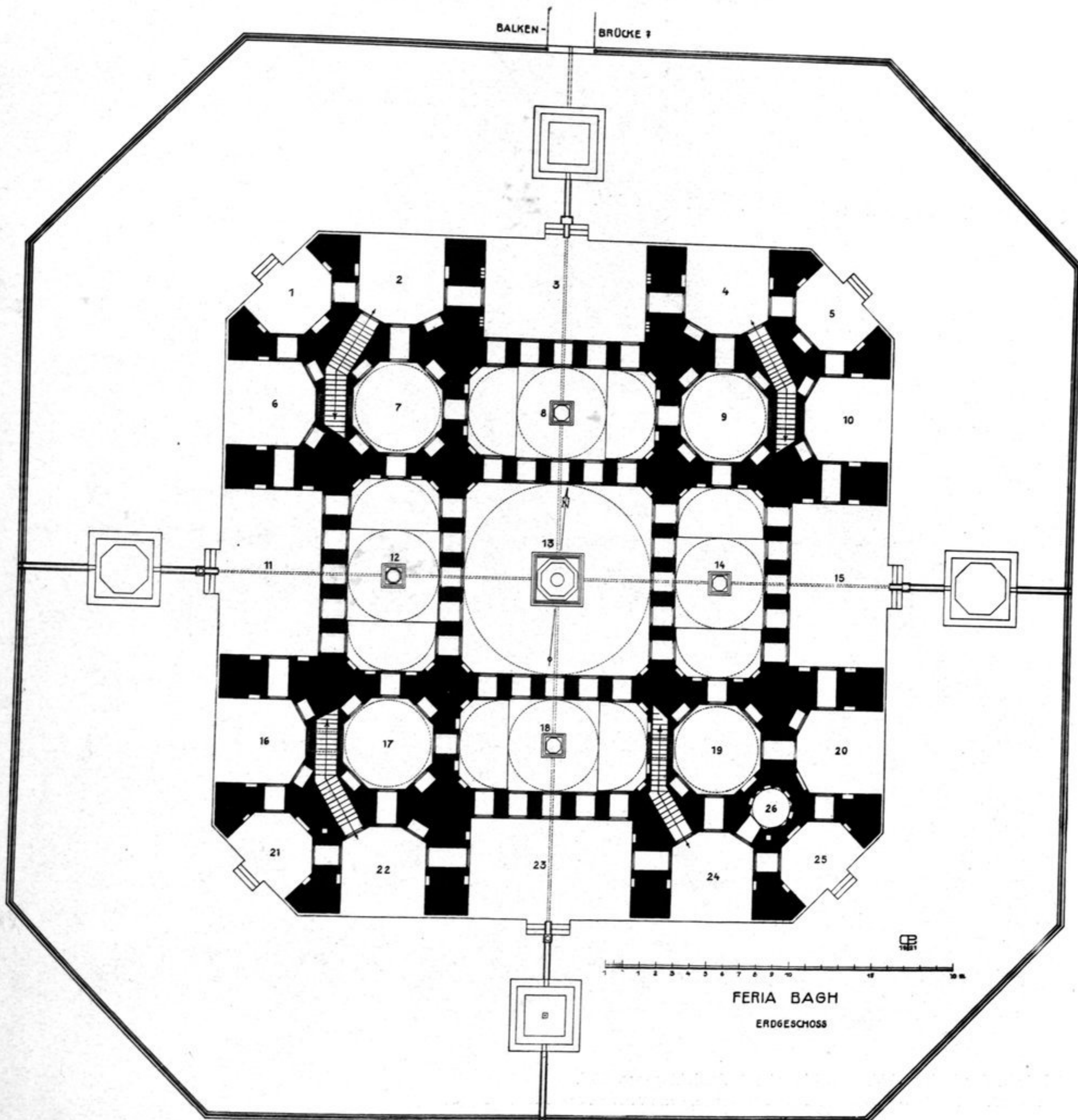
Grundriss des Erdgeschosses.
