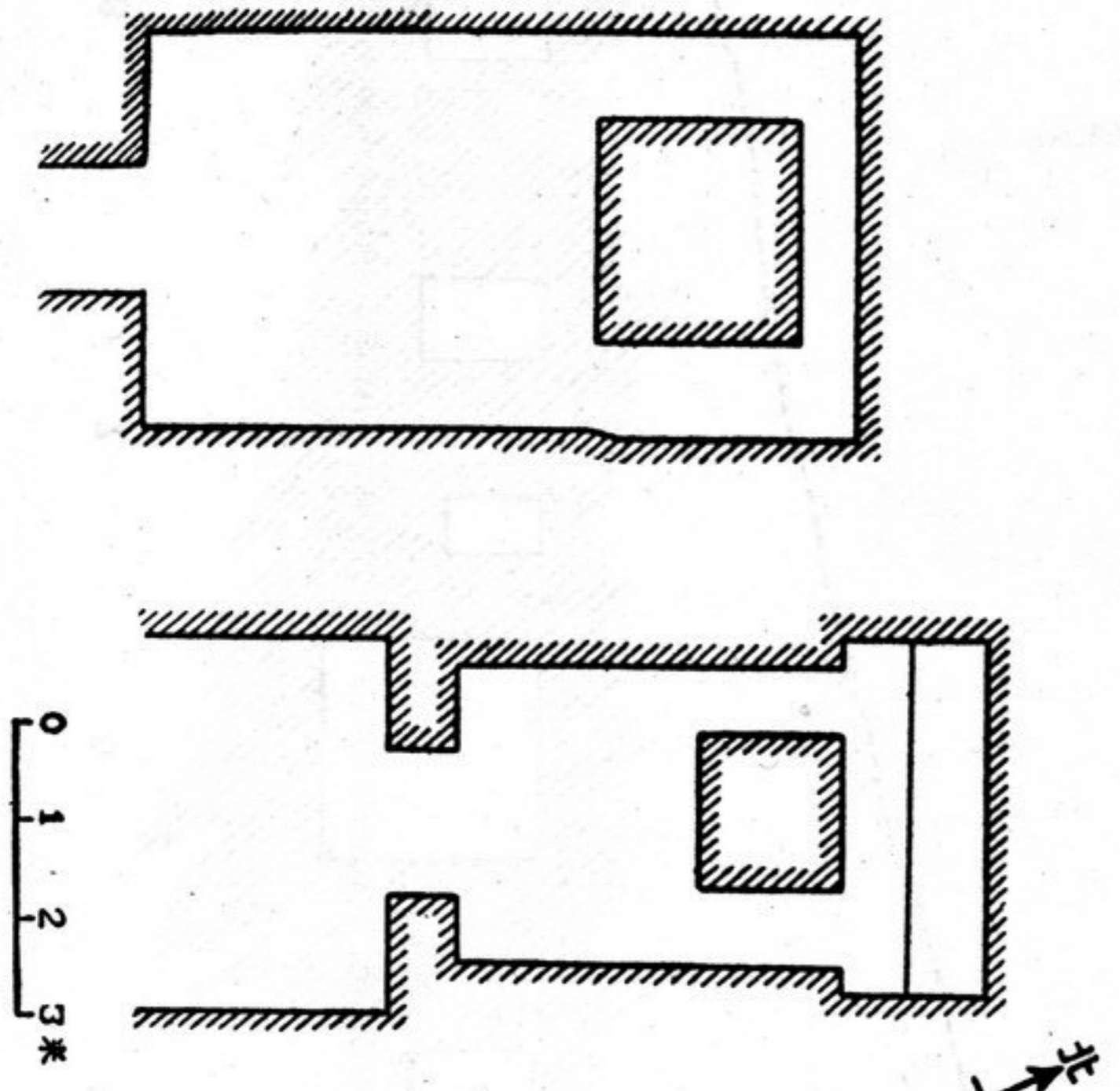
2. 克子爾明屋蘇格特溝西上層佛洞平面圖
