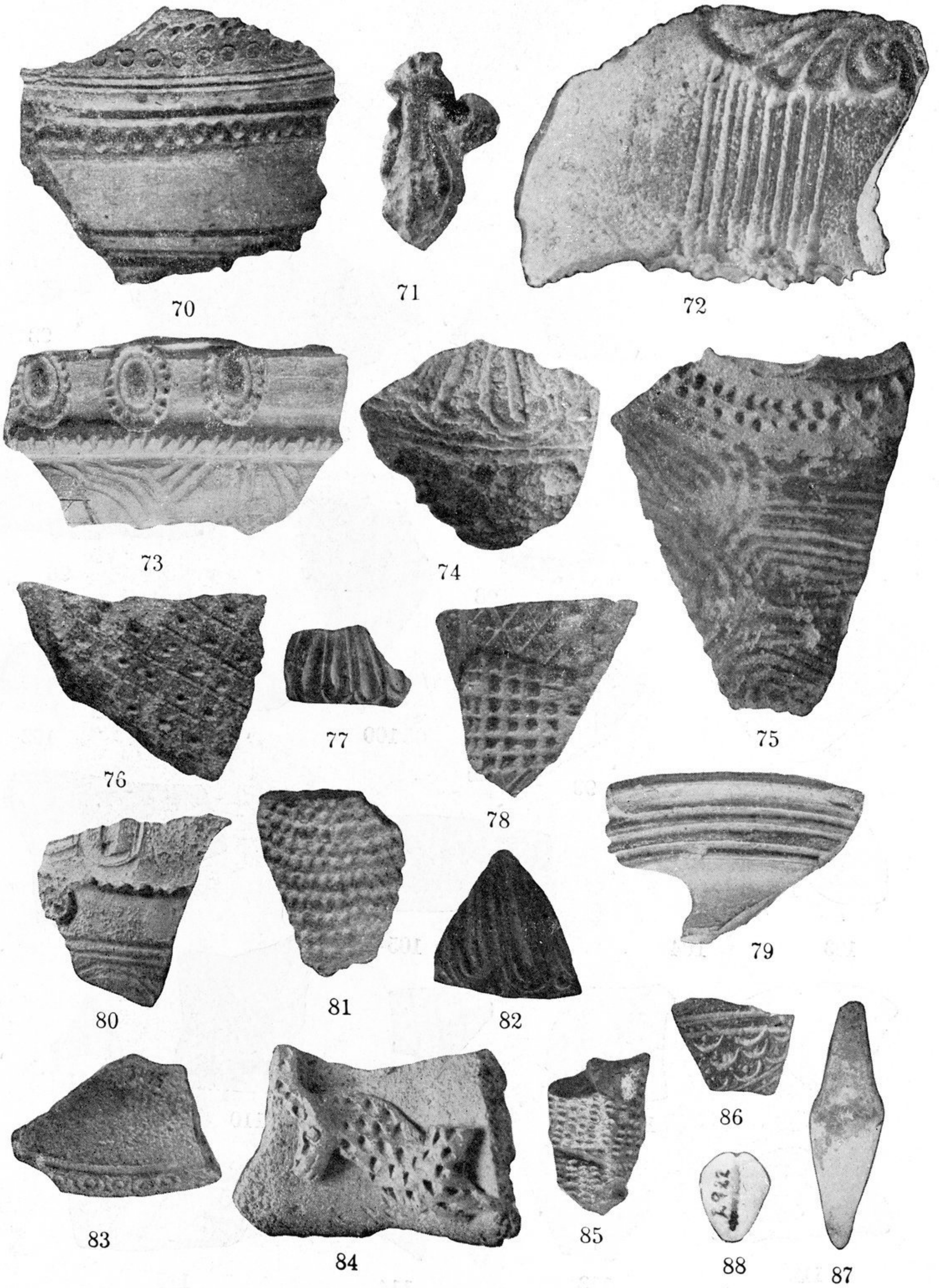
圖 70—86 剔紋紅陶片
