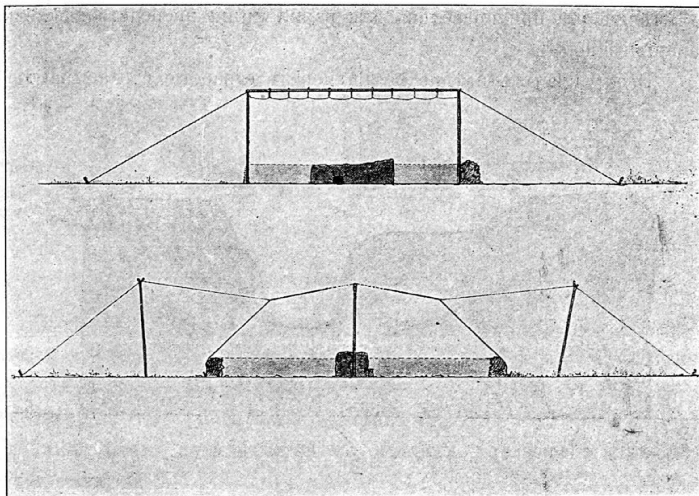
Тибетская палатка, въ разрѣзахъ продольномъ и поперечномъ.
