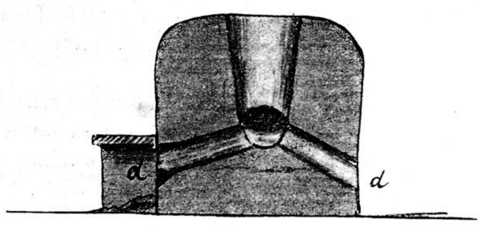
Поперечный разръзъ по линіи А—В.
