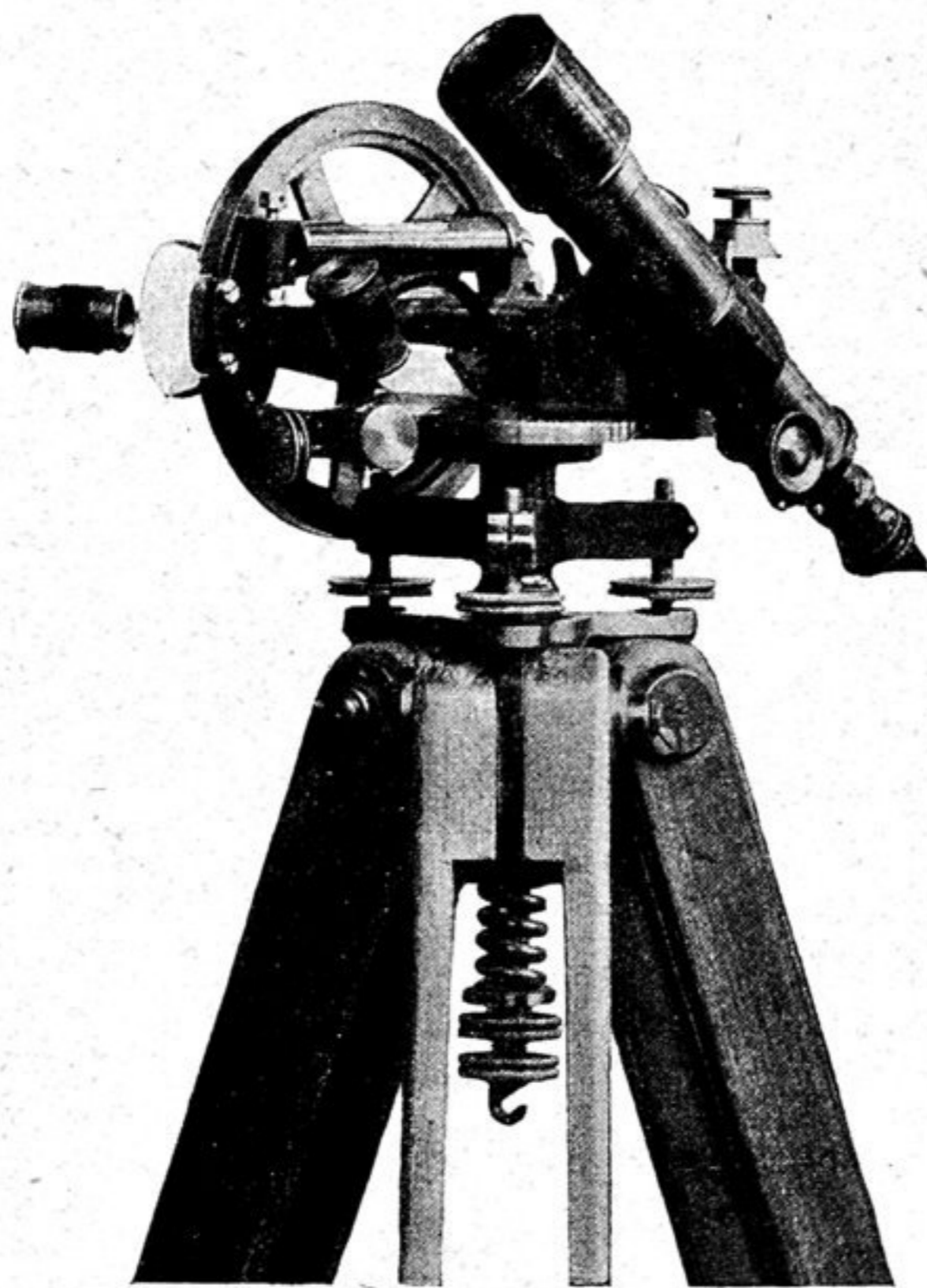
Универсальный инструментъ Гильдебрандта.
