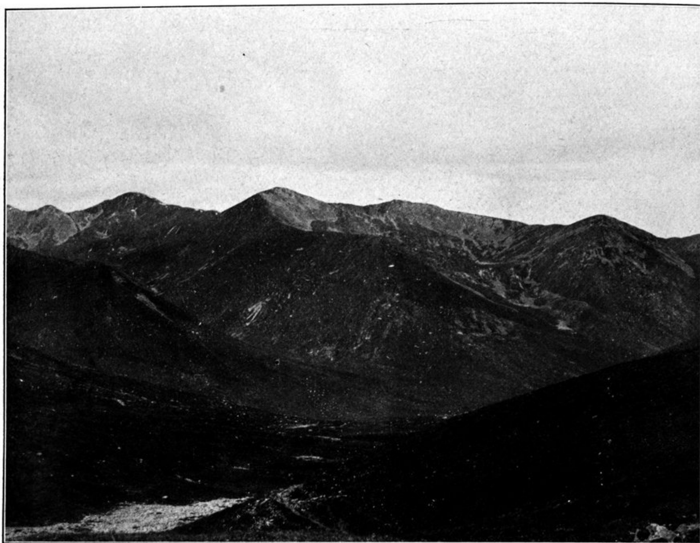
Karähnliche Talform in den Granitbergen von Ober-Zangskar (Somo).
