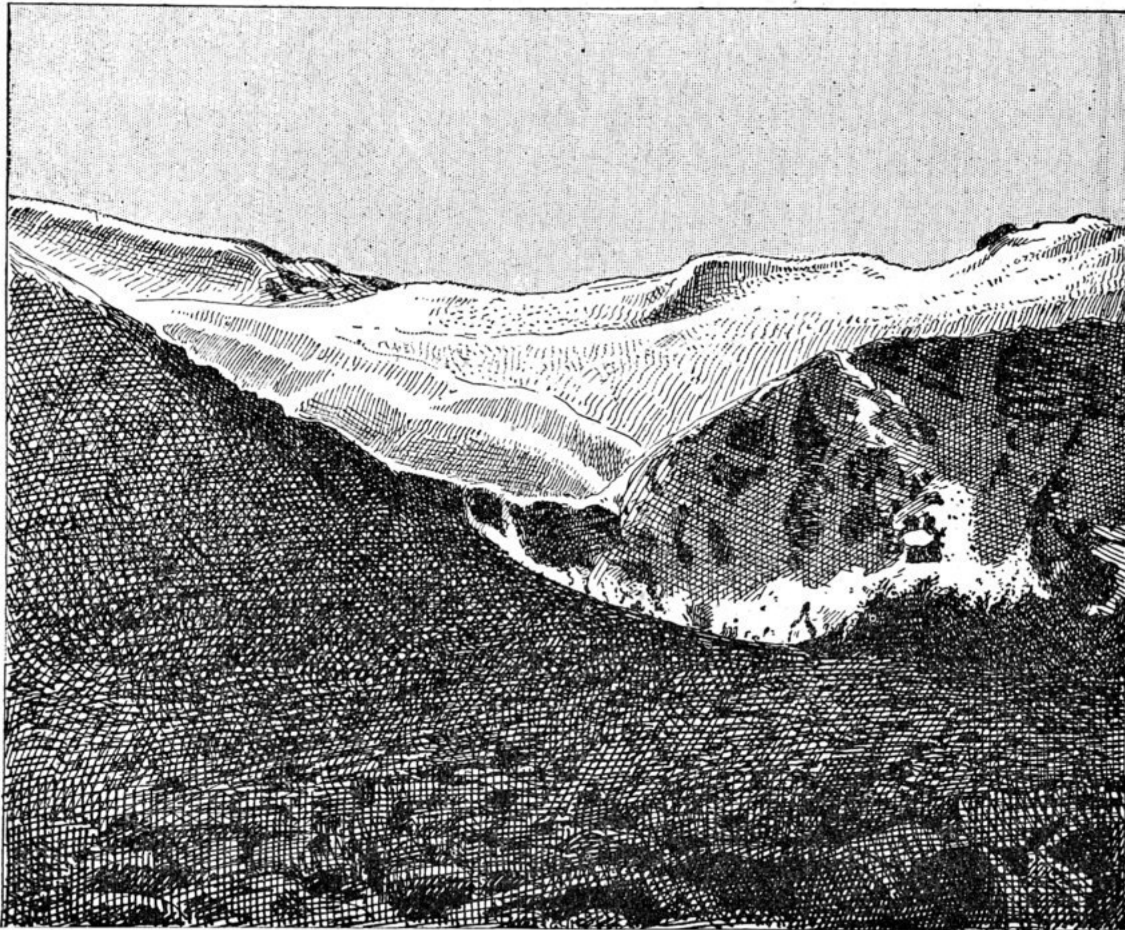
Glacier dans l'Oustoun tâgh entre le Karaoul davân et le Karakoram.
