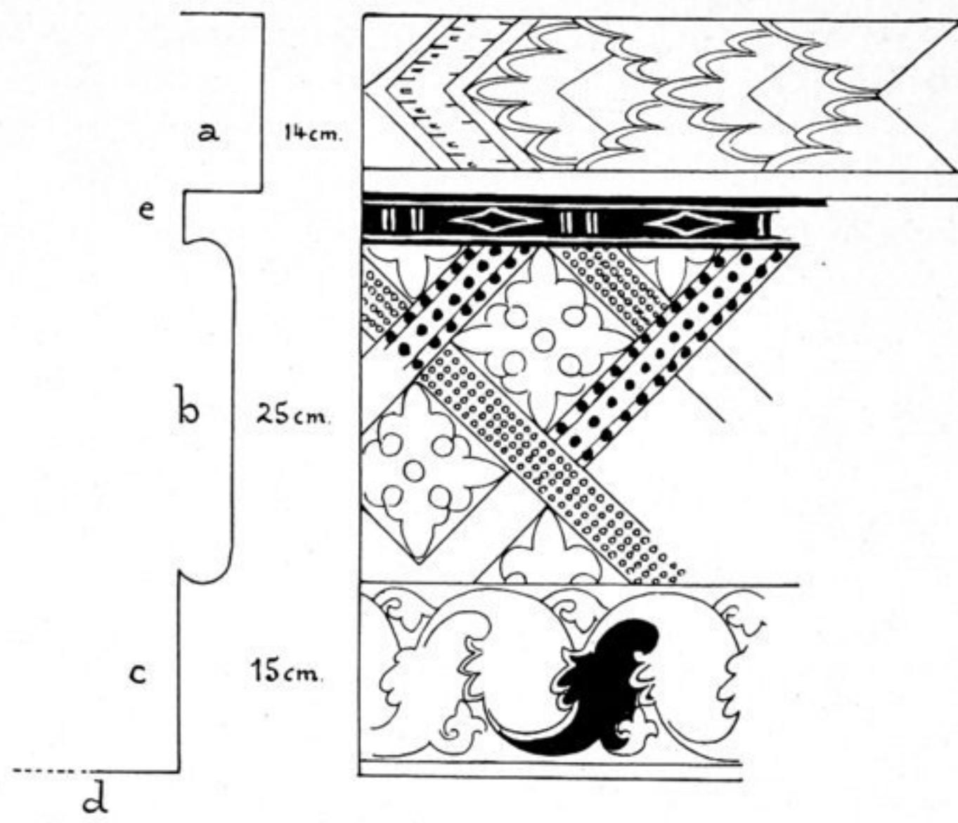
Fig. 186. Gesims unter der Decke, vgl. Fig. 184.
