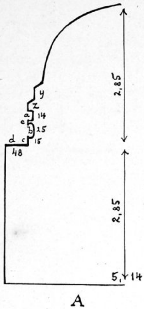
Fig. 184. Halber Durchschnitt der Haupthöhle A.
