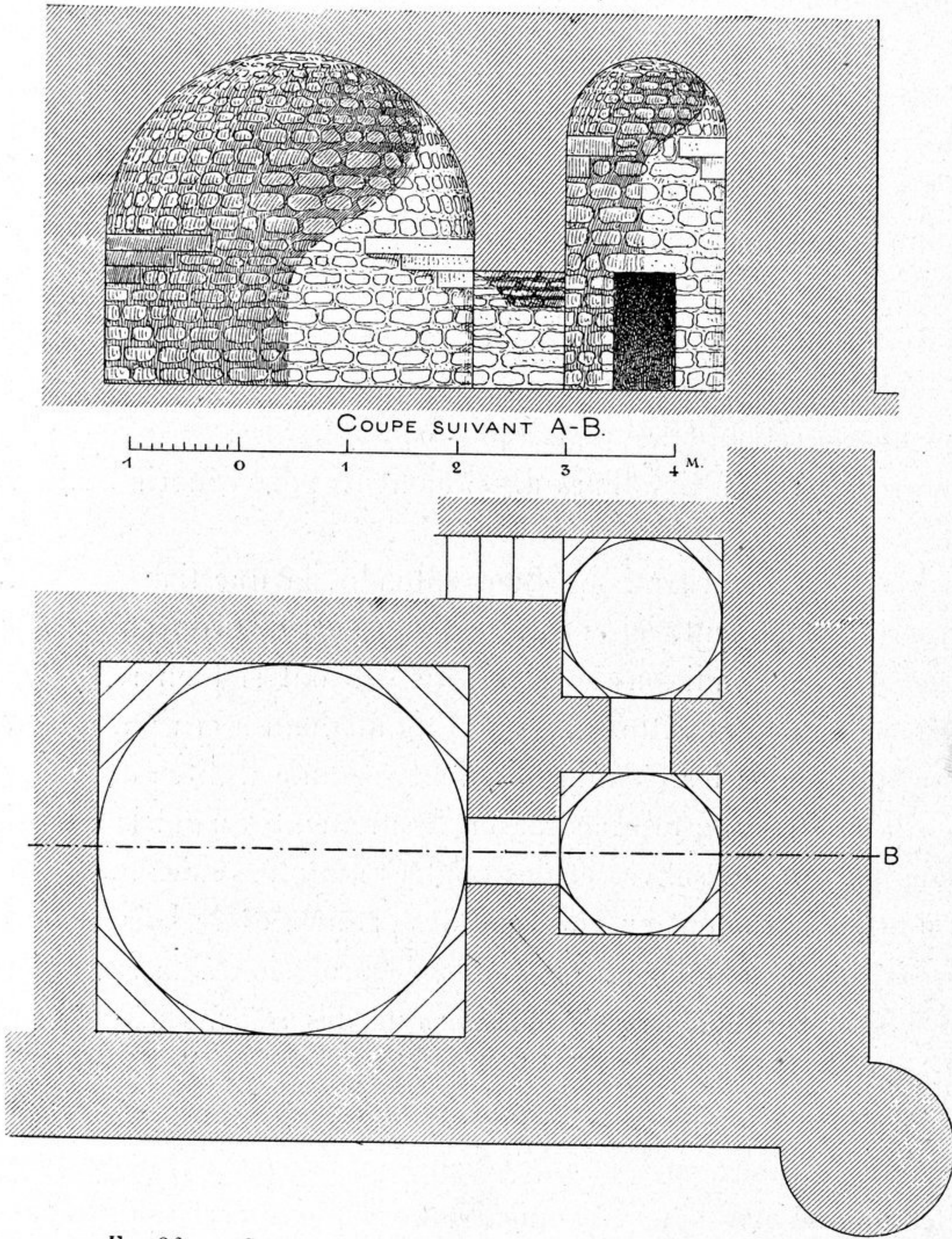
FIG. 36. — COUPOLES SUR SOUBASSEMENT CARRÉ : PLAN ET ÉLEVATION.
