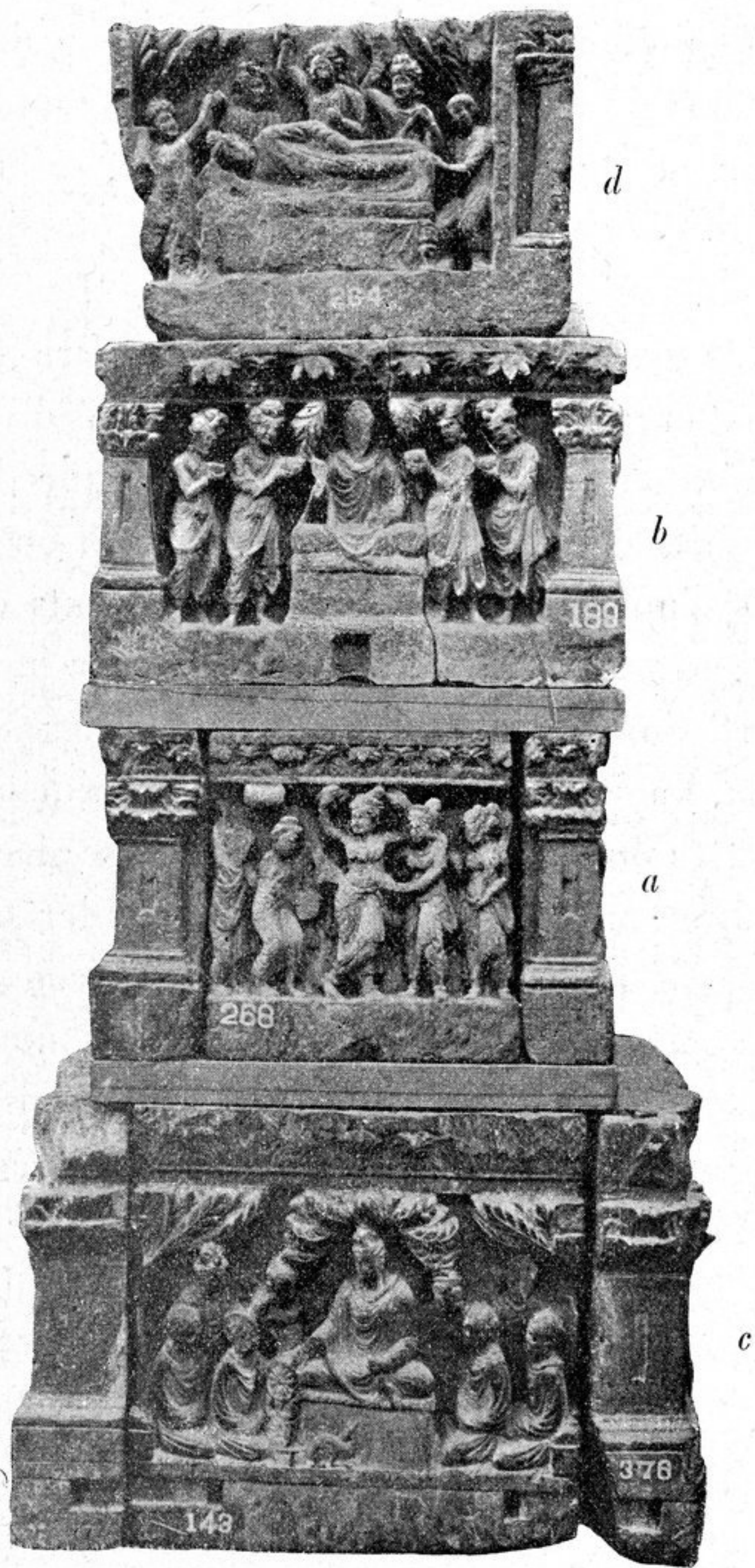
FIG. 208. — LES QUATRE GRANDES SCÈNES. Bases de stûpa, au Musée de Lahore.
